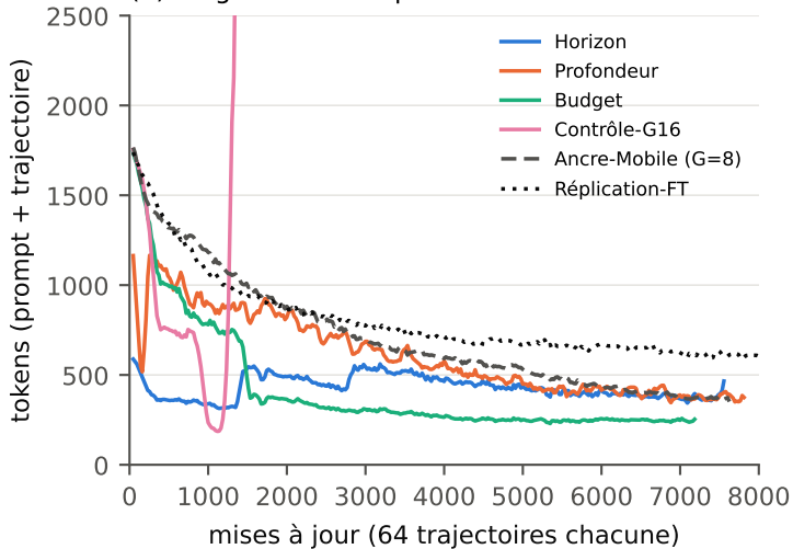
(a) longueur des séquences d'entraînement
