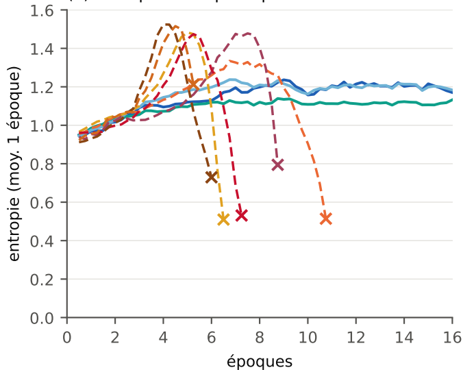
(a) entropie de la politique
