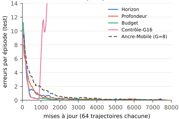
(a) erreurs de format par épisode
