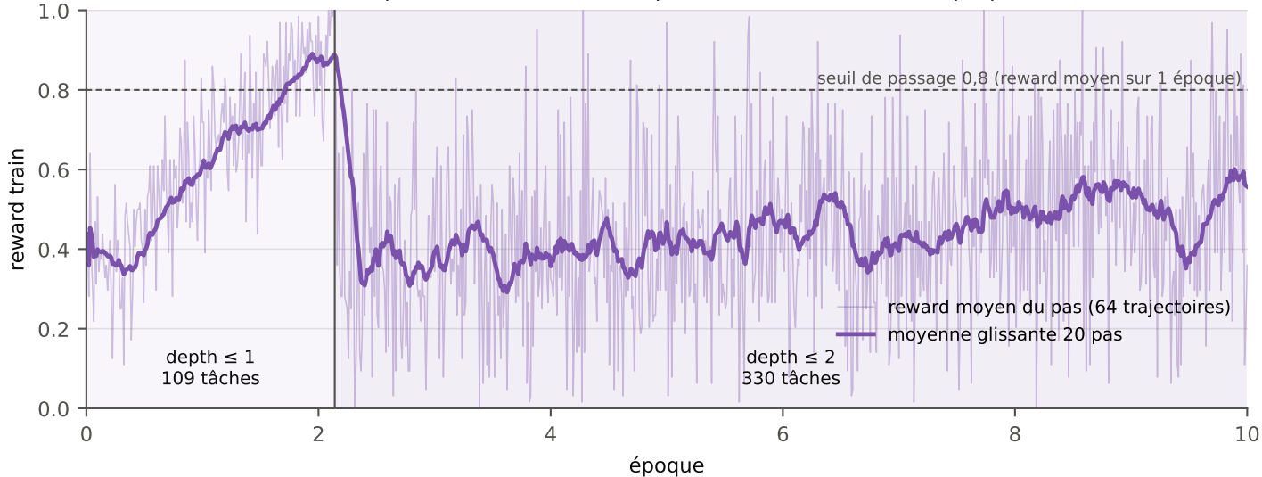
Curriculum Profondeur (exp33.1) : reward train et paliers auto-déclenchés, époques 0 à 10
