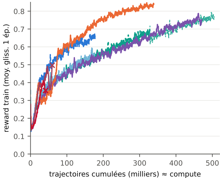
(d) reward train par trajectoires
