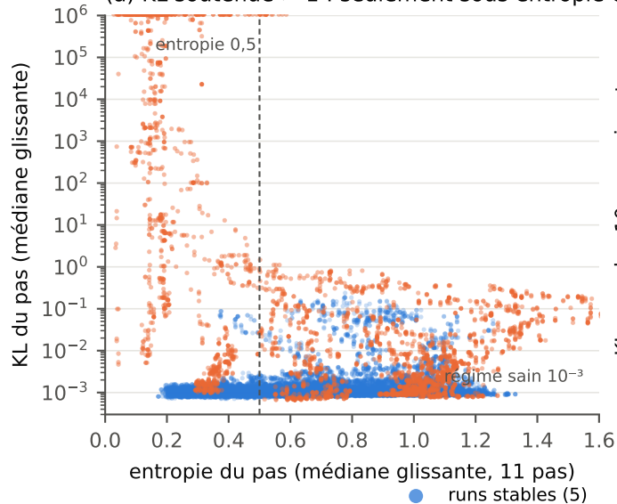
(a) KL soutenue > 1 : seulement sous entropie 0,5
