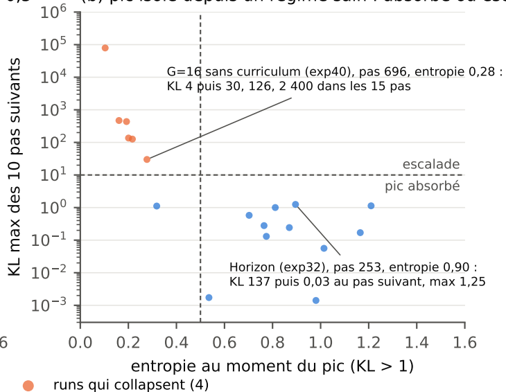
(b) pic isolé depuis un régime sain : absorbé ou escalade ?
