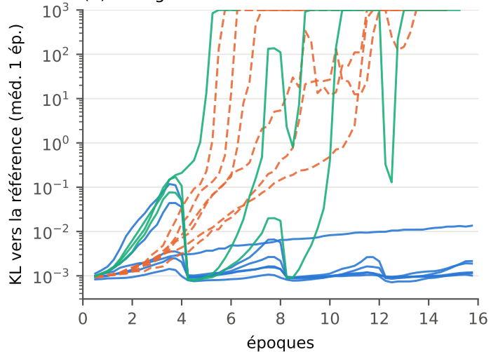
(b) divergence KL
