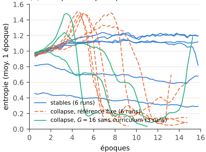
(a) entropie de la politique
