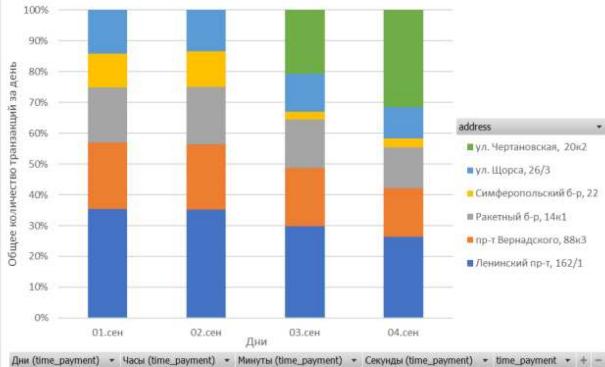
Доли транзакций по адресам в динамике за период
