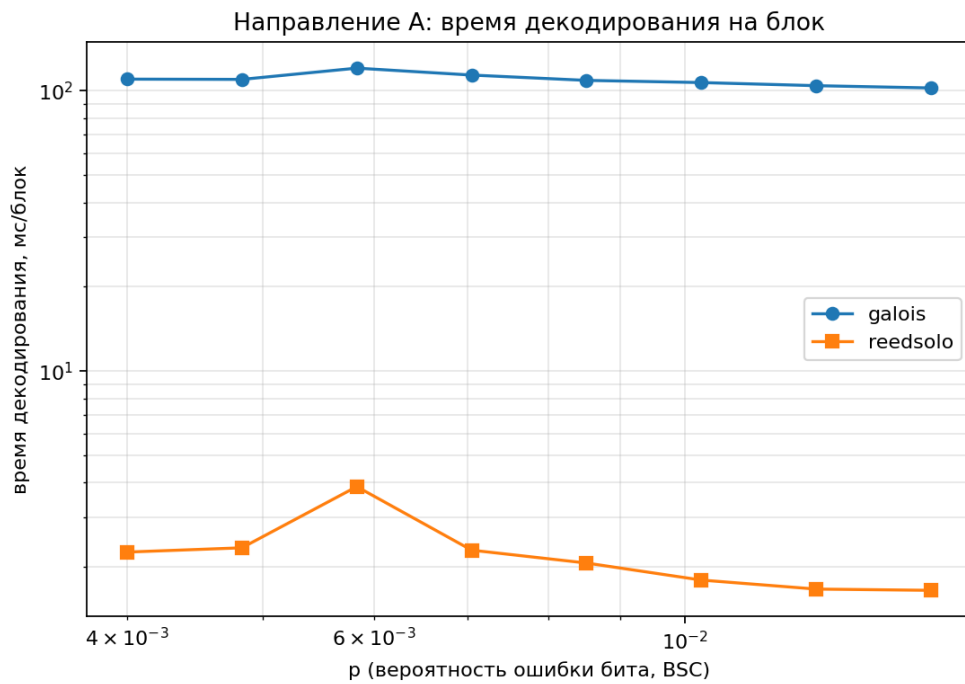
Рис. 3: Направление A: время декодирования на блок. reedsolo (нижняя кривая) на порядок быстрее galois (верхняя).
