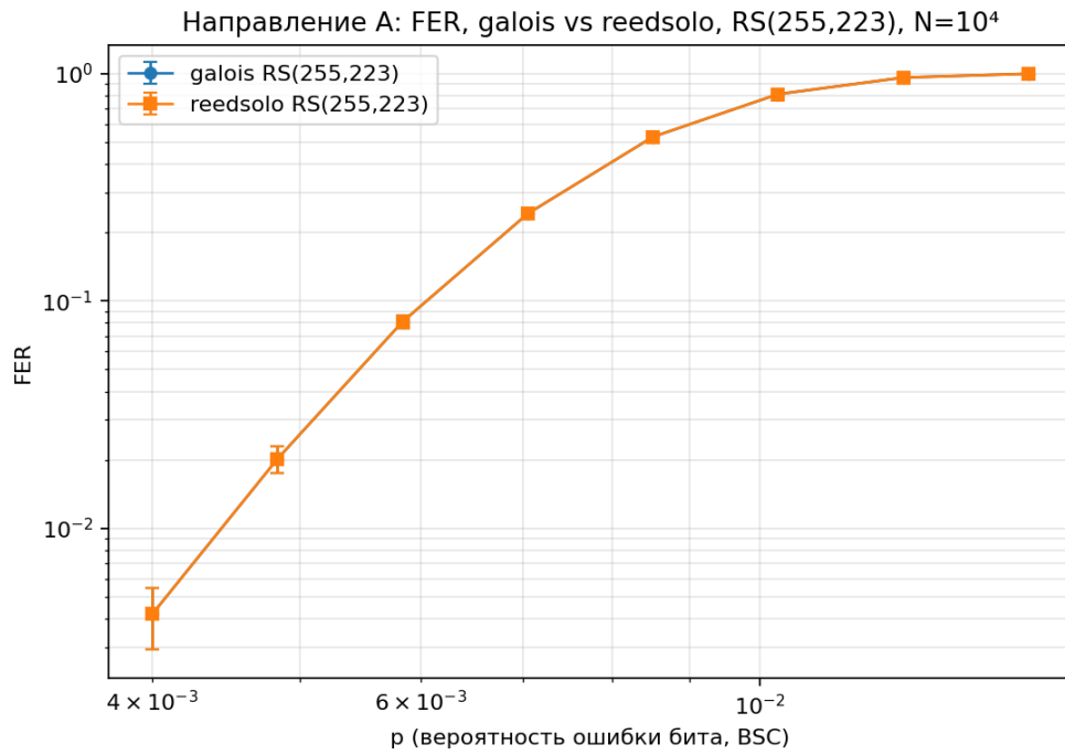
Рис. 2: Направление A: FER vs p . Кривые обеих библиотек полностью совпадают (маркеры наложены, доверительные интервалы перекрываются на 100%).
