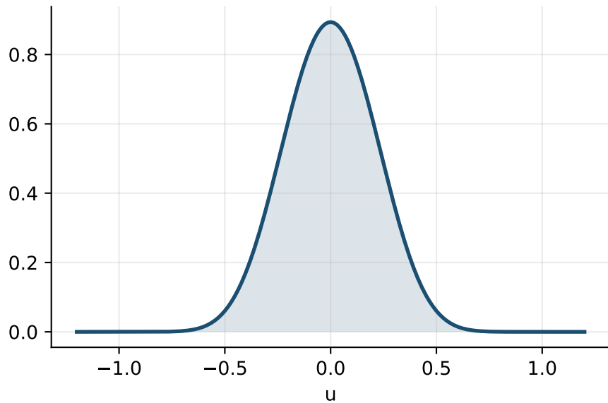
Pólya kernel \Phi(u)
