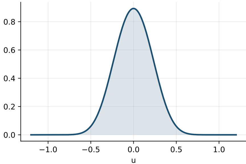
Pólya kernel \Phi(u)
