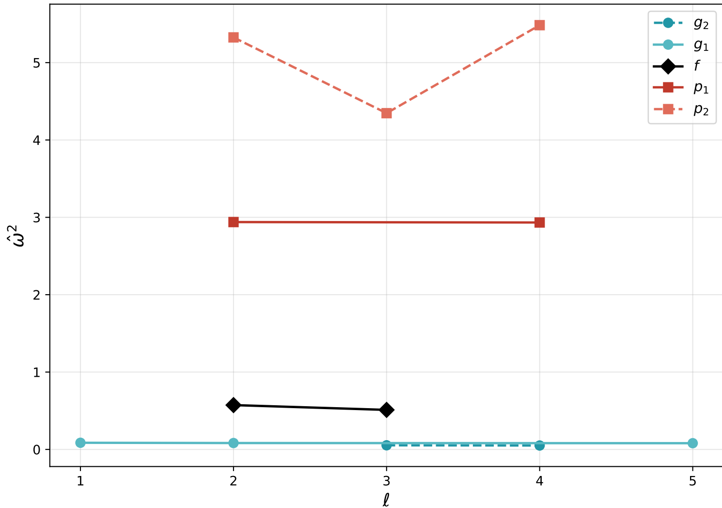
Ιδιοσυχνότητες πολυτροπικού αστέρα ( n = 1.5 , \gamma = 5/3 )
