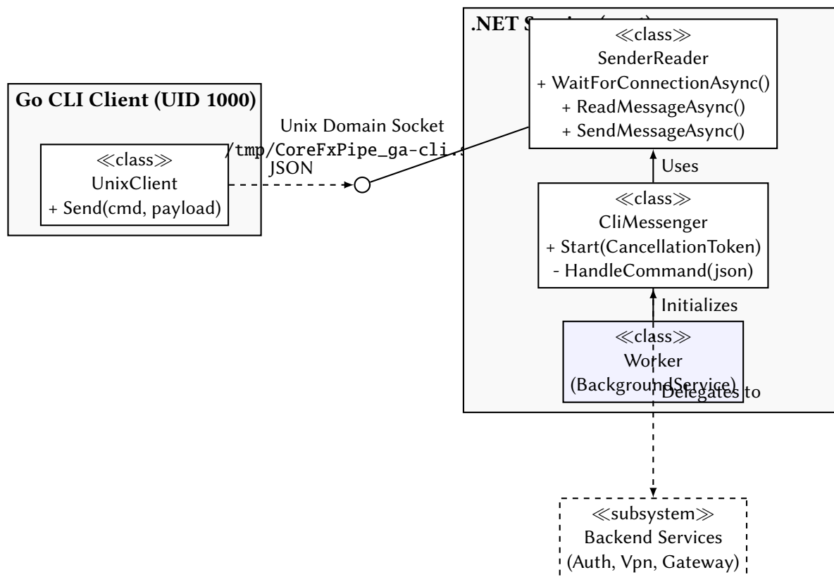
Obrázek 4.2.: Class diagram of IPC communication architecture.
