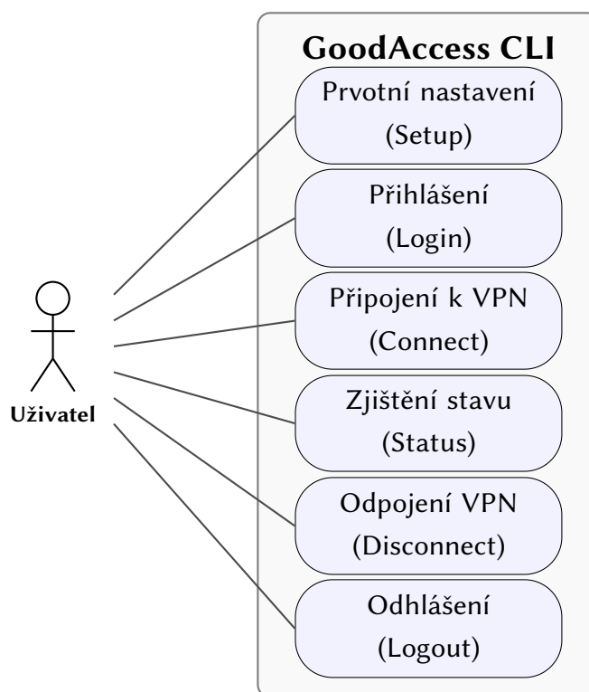
Obrázek 2.1.: Diagram případů užití GoodAccess CLI
