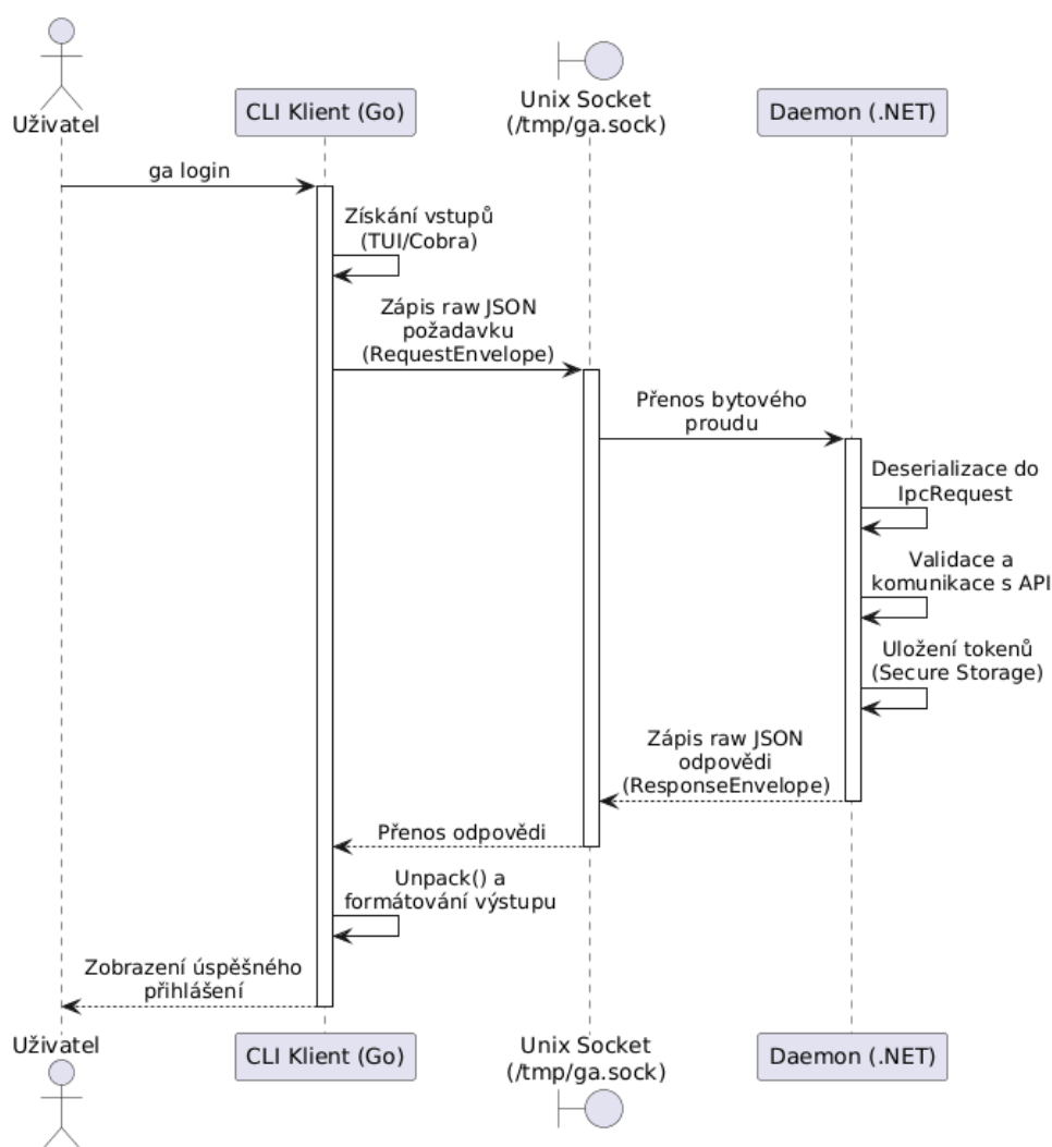
Obrázek 3.2.: Sekvenční diagram IPC komunikace při přihlášení.
