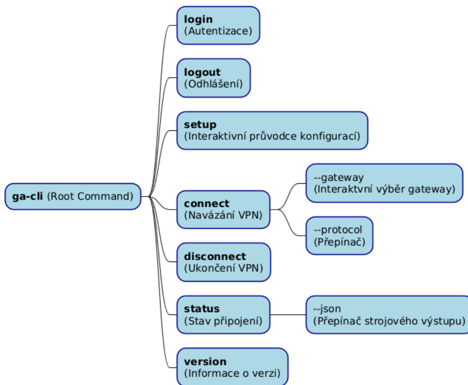
Obrázek 3.3.: Hierarchická struktura příkazů (Command Tree) aplikace ga-cli.
