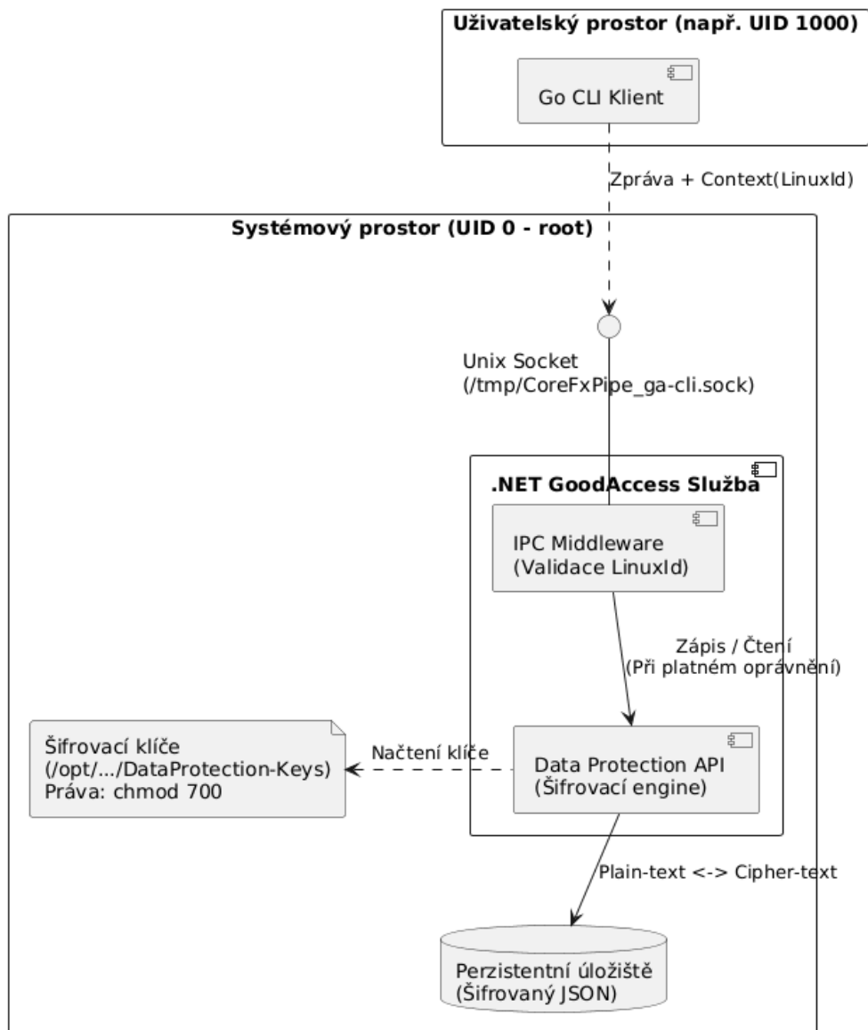
Obrázek 3.4.: Architektura zabezpečeného úložiště a správy klíčů
