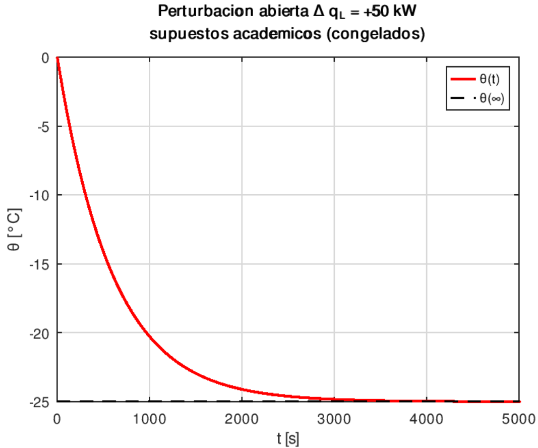
Figura 4. Respuesta abierta ante un incremento sostenido de carga de 50 kW.
