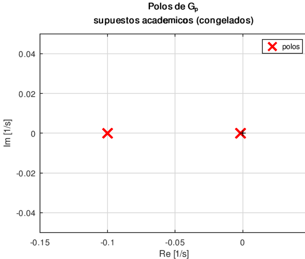
Figura 2. Polos del camino orden-temperatura.
