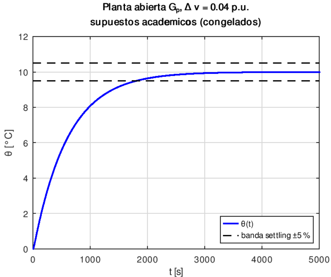
Figura 3. Respuesta abierta ante un incremento de orden de 0,04 p.u.
