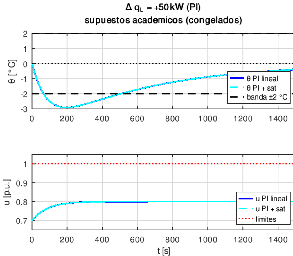
Figura 9. Rechazo de una perturbación sostenida de carga y acción de control.
