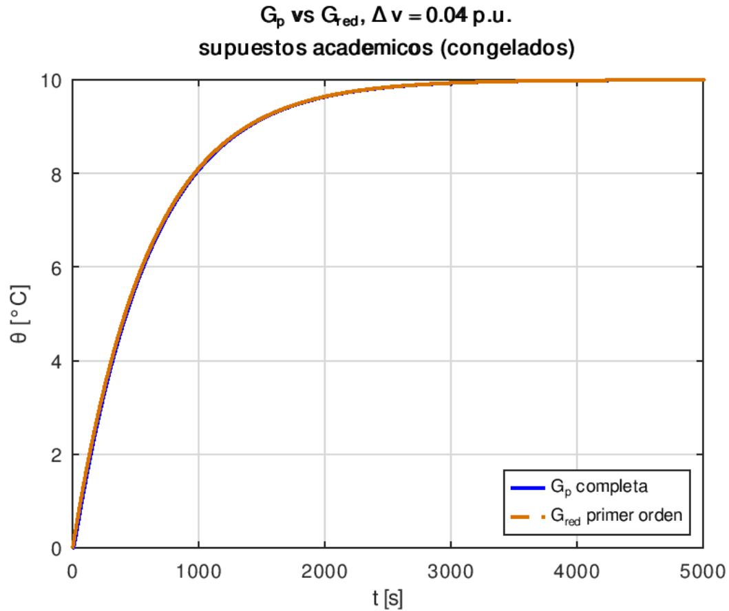
Figura 5. Comparación entre la planta completa y la aproximación dominante de primer orden.
