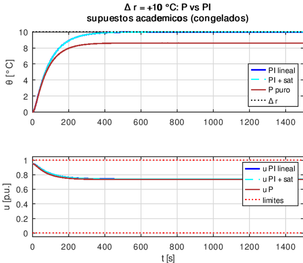
Figura 8. Seguimiento de referencia y acción de control para P y PI.
