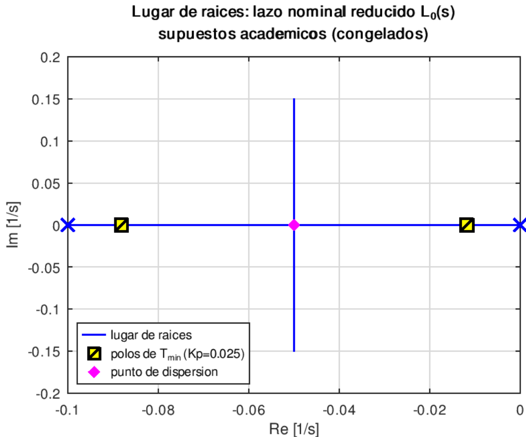
Figura 6. Lugar de raíces del lazo nominal reducido y ubicación de los polos adoptados.
