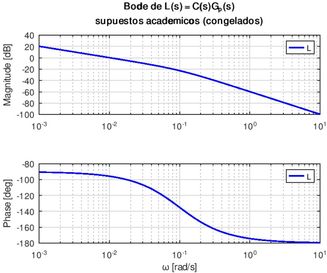
Figura 7. Respuesta frecuencial del lazo abierto compensado.
