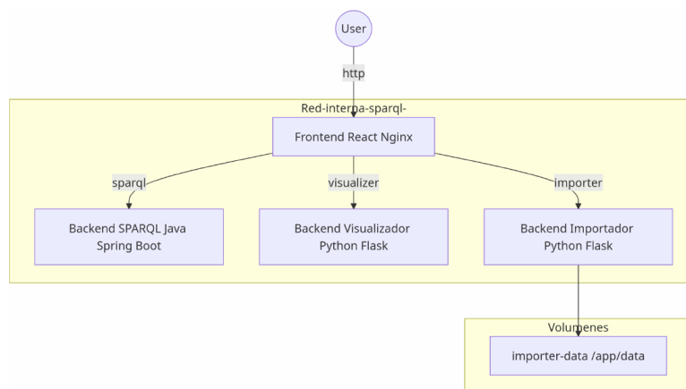
Figura 40: Diagrama de despliegue de la aplicación con docker compose
