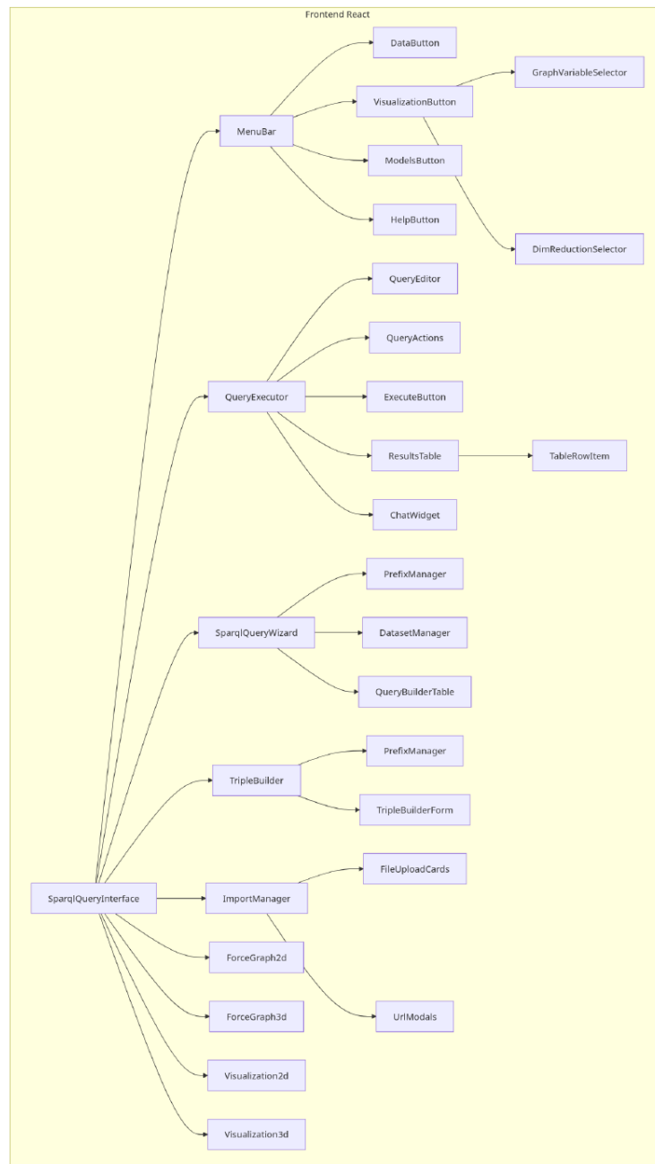
Figura 38: Jerarquía de componentes del frontend
