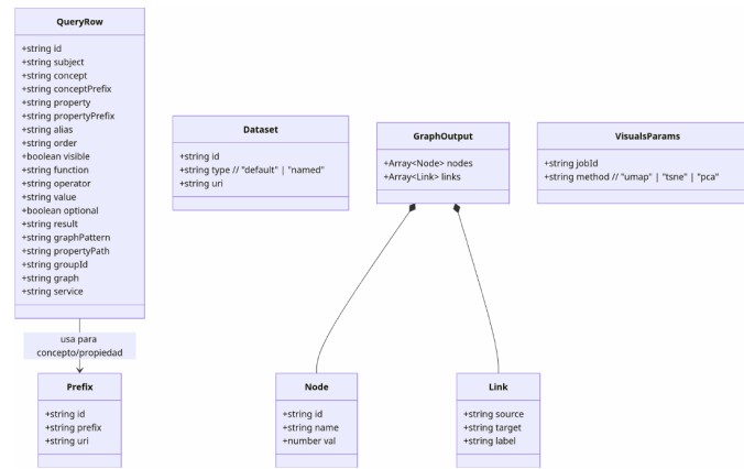
Figura 39: Diagrama de entidades principales del frontend
