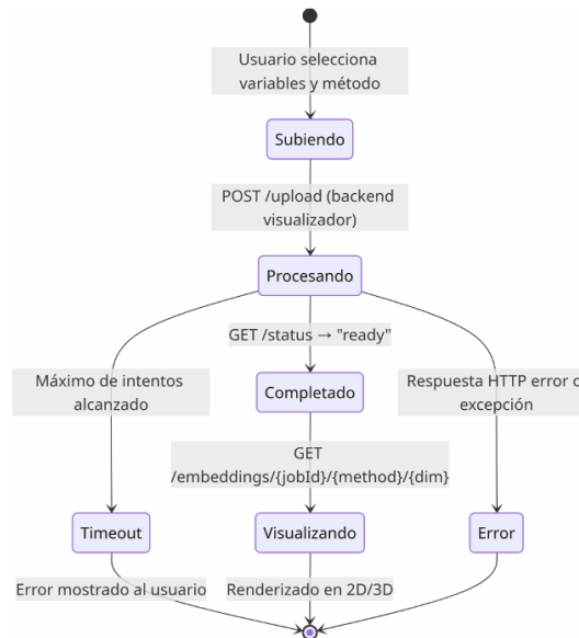
Figura 37: Diagrama de estados del servicio de visualización
