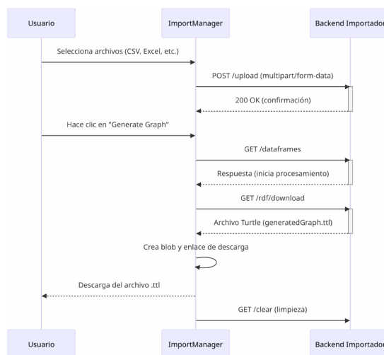
Figura 18: Diagrama secuencia Visualización de grafo
