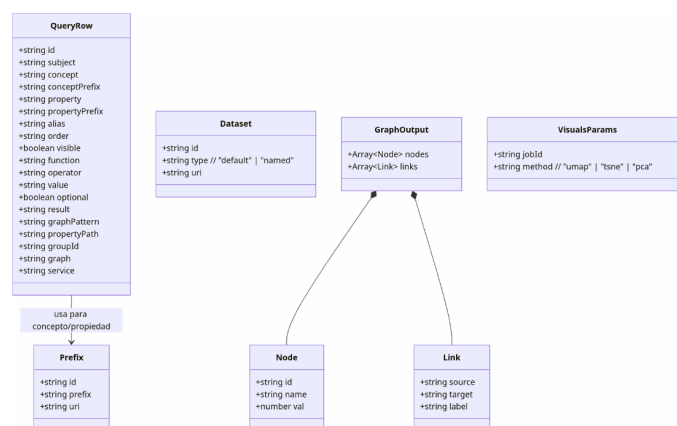
Figura 8: Diagrama de entidades principales del frontend
