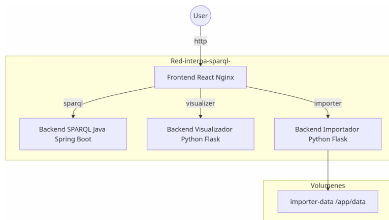
Figura 9: Diagrama de despliegue de la aplicación con docker compose
