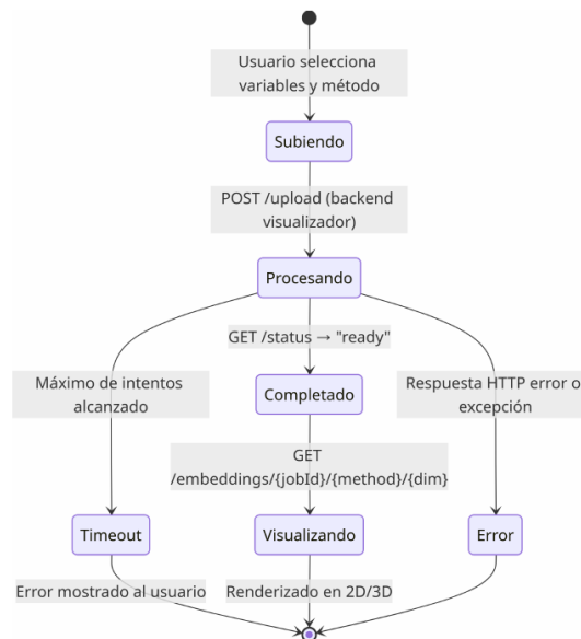
Figura 6: Diagrama de estados del servicio de visualización
