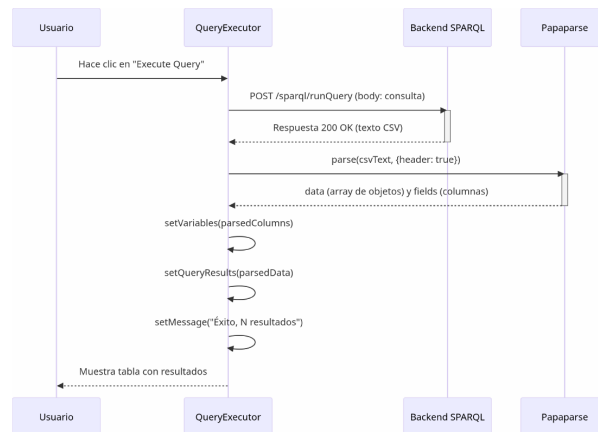
Figura 1: Diagrama secuencia ejecución de una consulta
