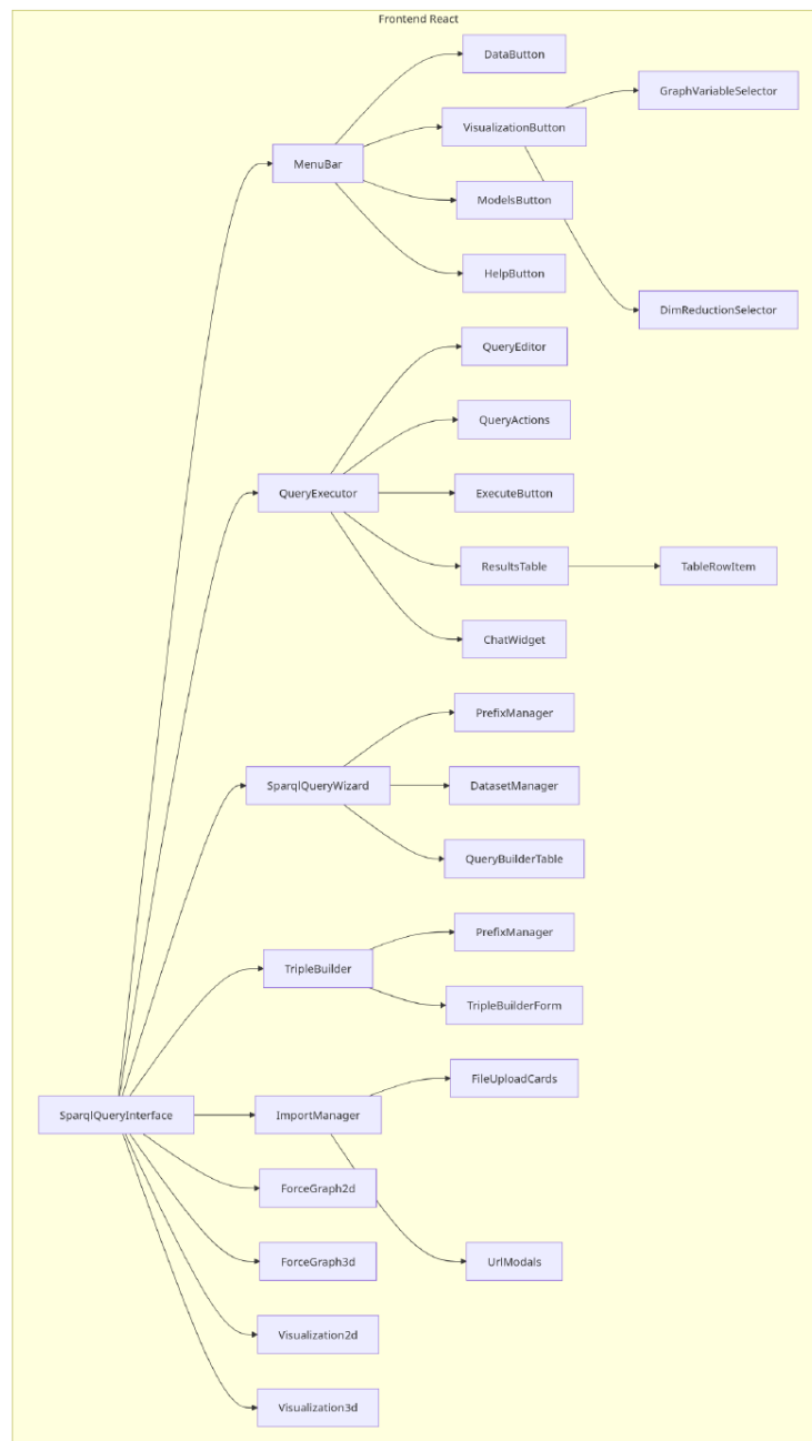
Figura 7: Jerarquía de componentes del frontend
