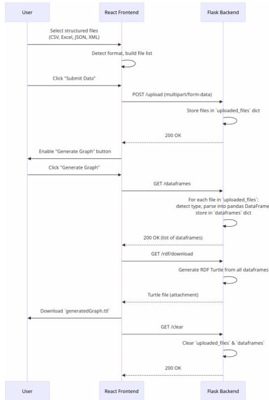
Figura 4: Diagrama de secuencia para usar el microservicio de importacion
