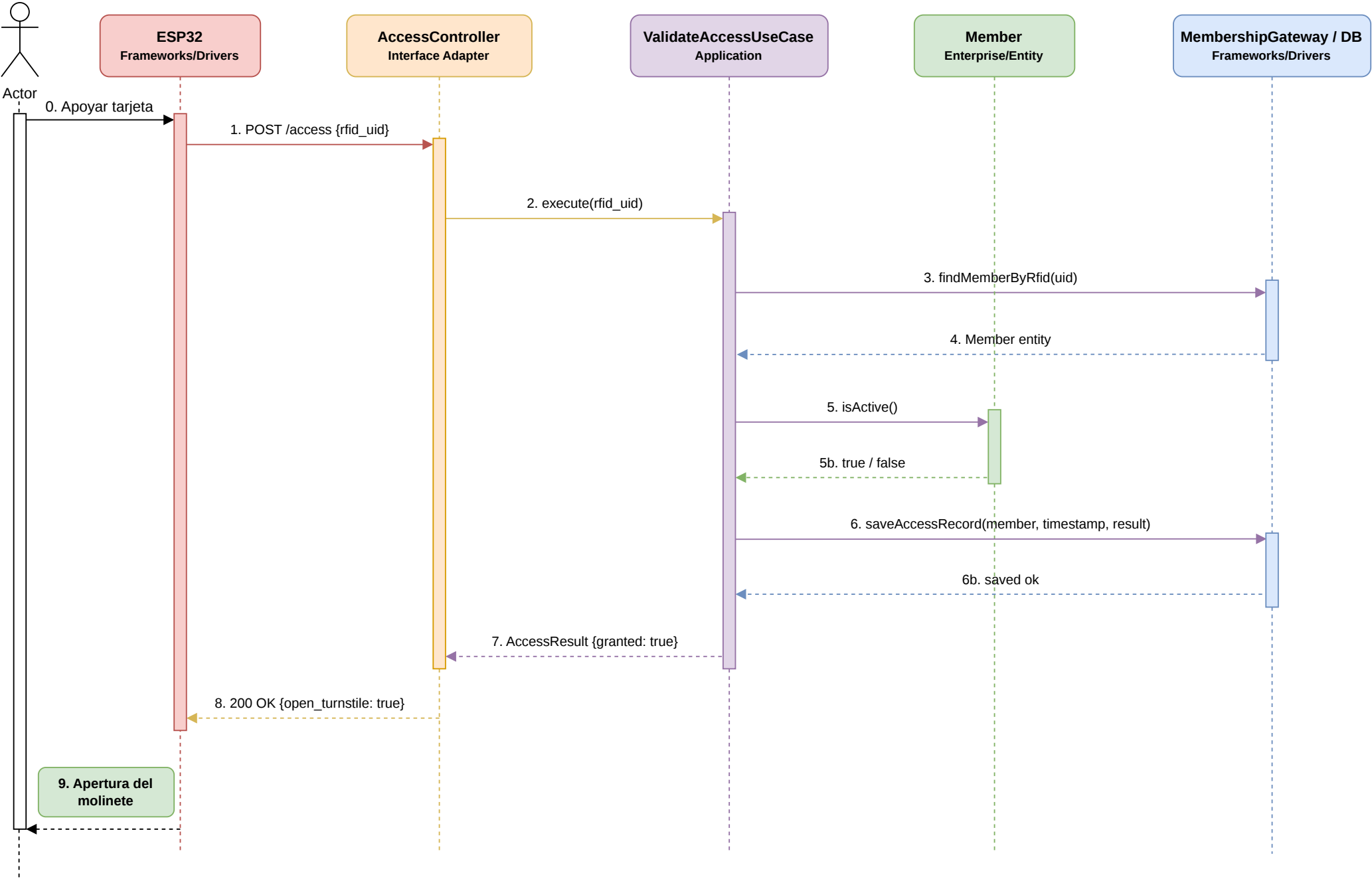
Diagrama de Secuencia — Validar Ingreso RFID (Clean Architecture)
