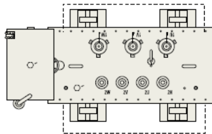
Transformadores Subtransmisión - Relación 33000 +2,5%0;-3x2,5% / 13860 V/V
