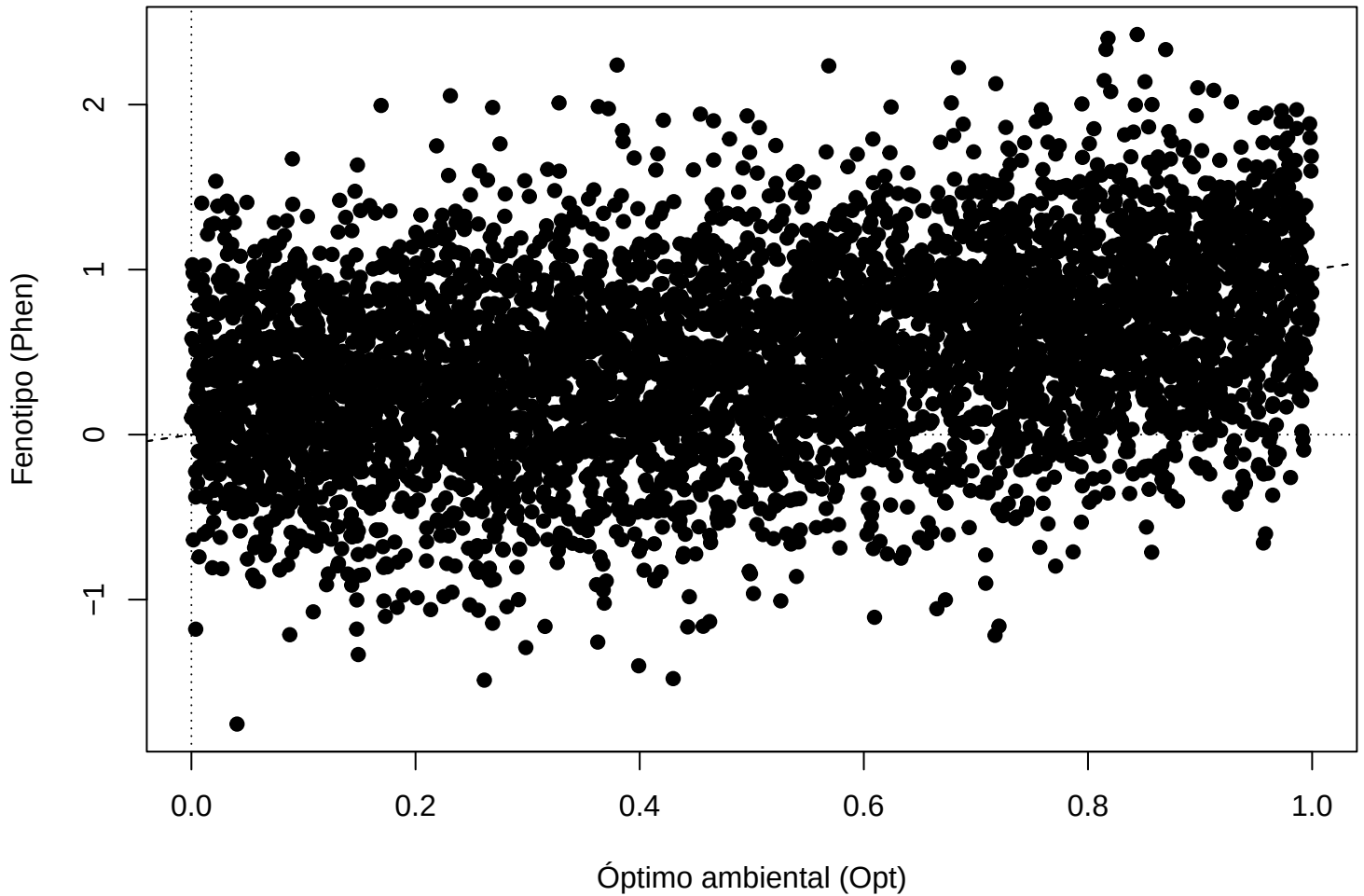
Fenotipo vs. Óptimo ambiental h^2 = 0.5
