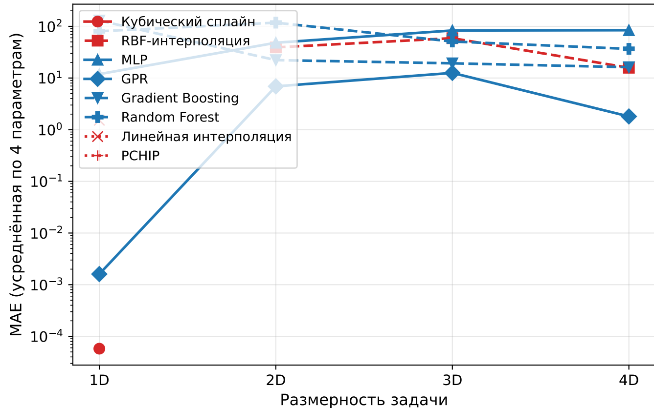
Точность методов при росте размерности
