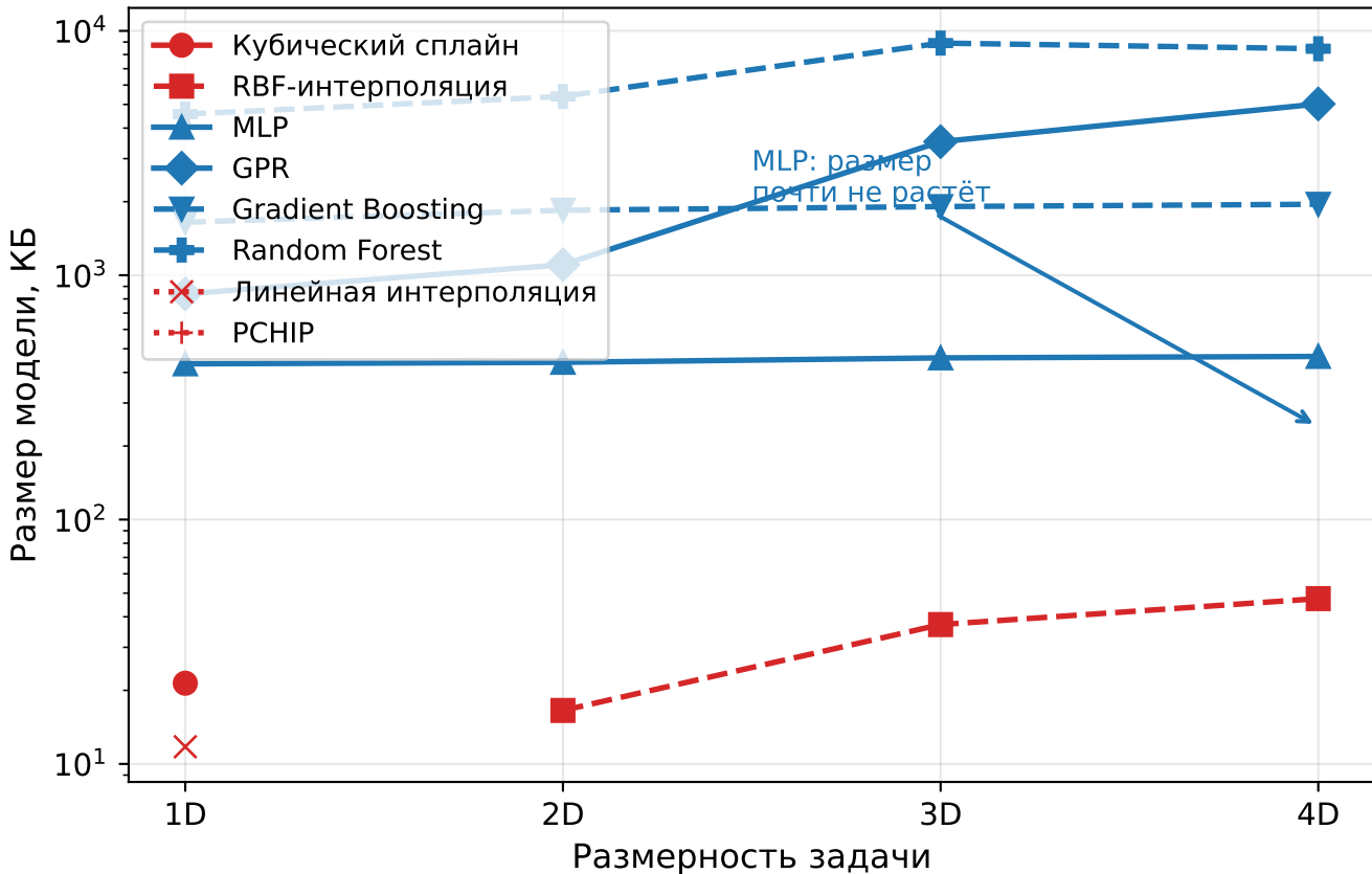
Рост размера модели при увеличении размерности
