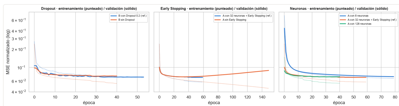
Figura 11. Curvas de entrenamiento (punteadas) y validación (sólidas) de los experimentos de Dropout, Early Stopping y número de neuronas.
