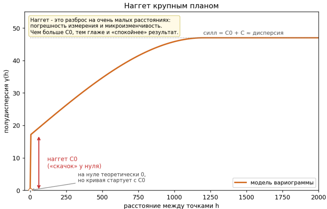
Рис. 6: Наггет крупным планом: модель стартует у нуля не с 0, а со «скачка» C0. Это разброс на сверхмалых расстояниях (погрешность измерения, микроизменчивость). Полка C0 + C \approx дисперсии данных.
