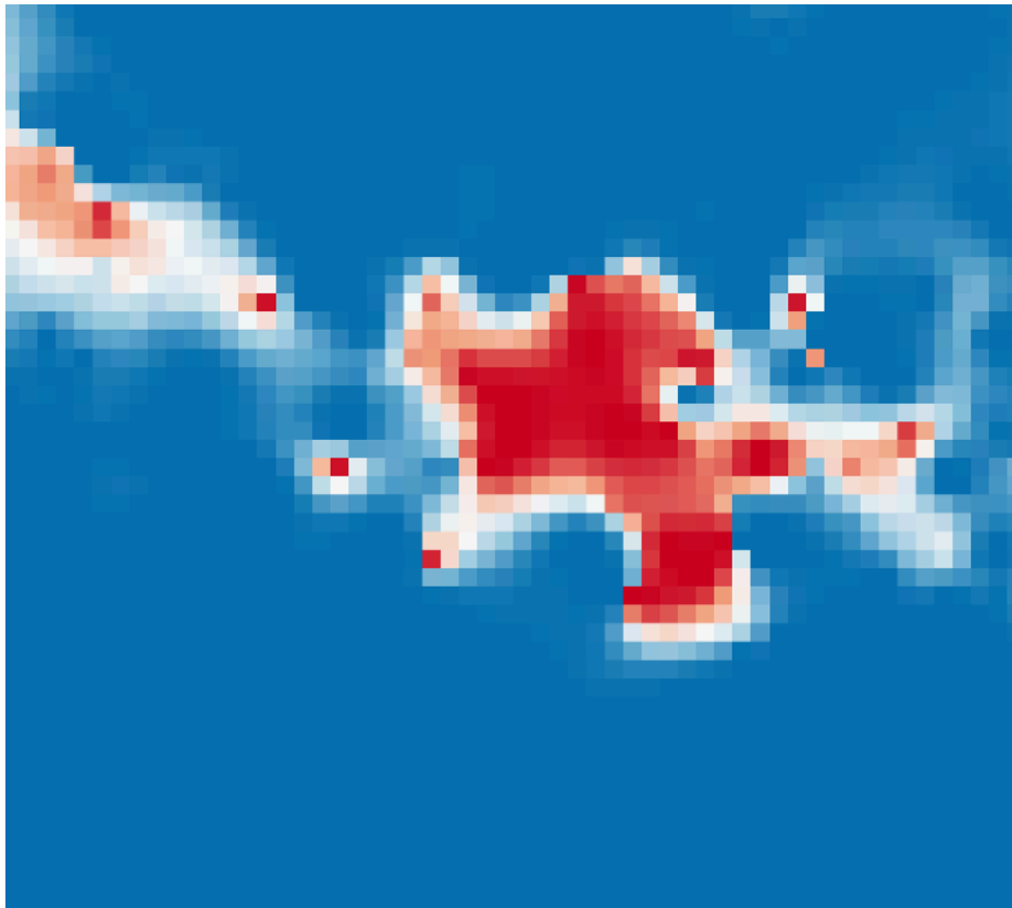
Рис. 26: Карта вероятности превышения с расходящейся шкалой и переломом на 0.5. Красное - значение уверенно выше порога, синее - уверенно ниже, белый поясok по линии P=0.5 - зона неопределённости (спорные значения). Чем дальше от скважин, тем шире поясok.
