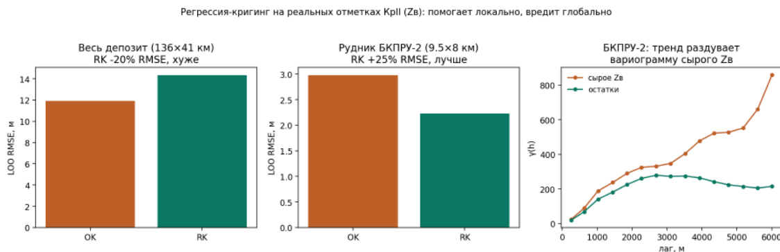
Рис. 11: Снятие тренда на реальных данных: поверхность пласта с выраженным региональным падением. Тренд снят полиномом, кригованы остатки, тренд возвращён к оценке.
