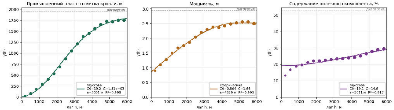
Рис. 13: Три типа параметров одного пласта в едином окне: отметка кровли (почти нулевой наггет, гладкая поверхность), мощность (наггет около трети, сферическая) и содержание (наггет сопоставим со вкладом, шумный параметр).
