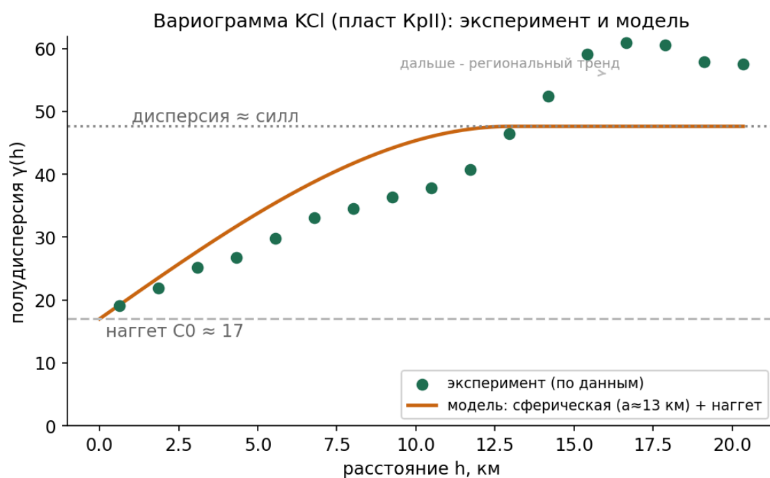
Рис. 8: Экспериментальная вариограмма KCl по пласту КрII и подобранная модель: наггет C_0 \approx 17 , силл совпал с дисперсией данных, радиус \approx 13 км. Точки дальше силла - региональный тренд.
