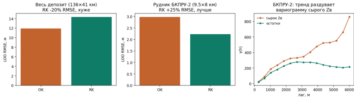
Рис. 11: Снятие тренда на реальных данных: поверхность пласта с выраженным региональным падением. Тренд снят полиномом, кригованы остатки, тренд возвращён к оценке.
