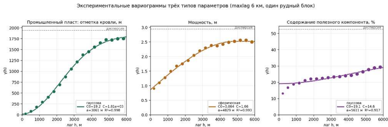
Рис. 13: Три типа параметров одного пласта в едином окне: отметка кровли (почти нулевой наггет, гладкая поверхность), мощность (наггет около трети, сферическая) и содержание (наггет сопоставим со вкладом, шумный параметр).
