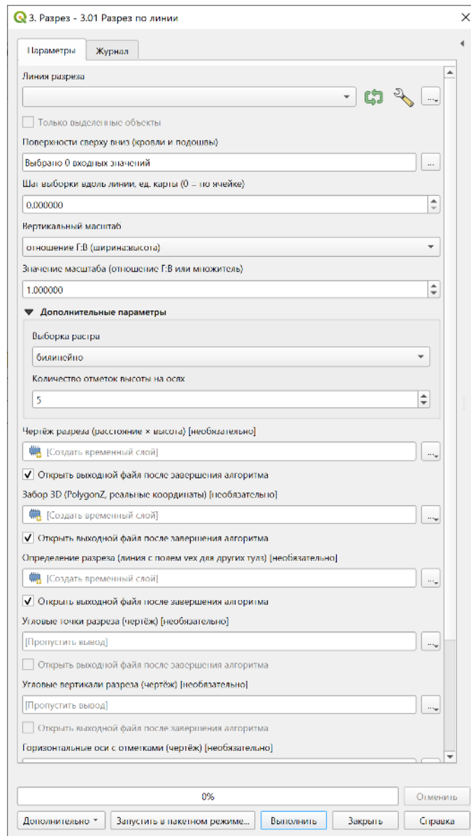
Рис. 36: Окно 3.01: линия разреза, поверхности сверху вниз, вертикальный масштаб и выходы чертежа.
