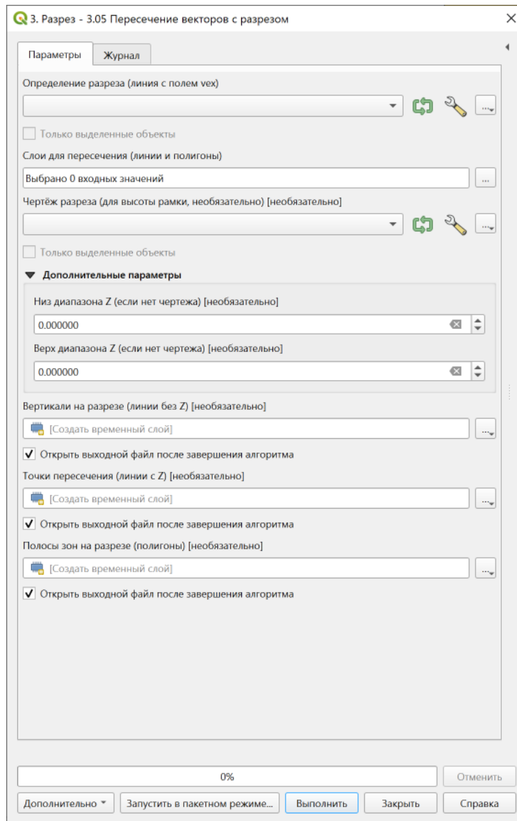
Рис. 41: Окно 3.05: слой для пересечения, чертёж разреза и три выхода (вертикали, точки, полосы зон).
