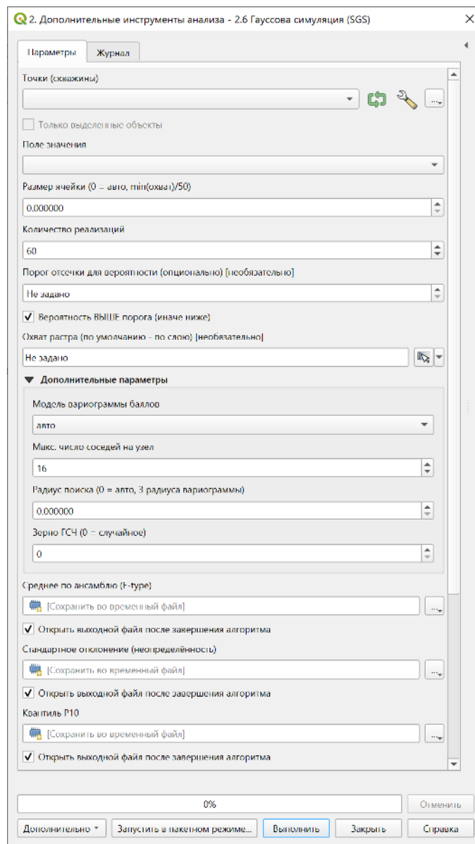
Рис. 35: Окно 2.6: точки, поле значения, количество реализаций и доп-параметры симуляции.
