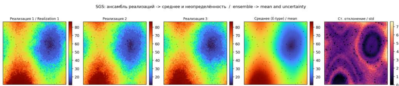
Рис. 34: Ансамбль реализаций SGS и производные от него среднее и неопределённость.
