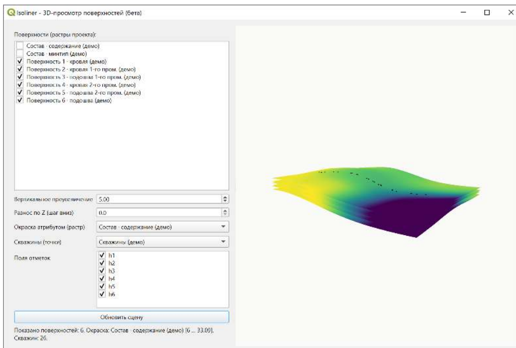
Рис. 45: Этажерка поверхностей, окрашенных атрибутивным гридом; шкала с диапазоном - под кнопками.
