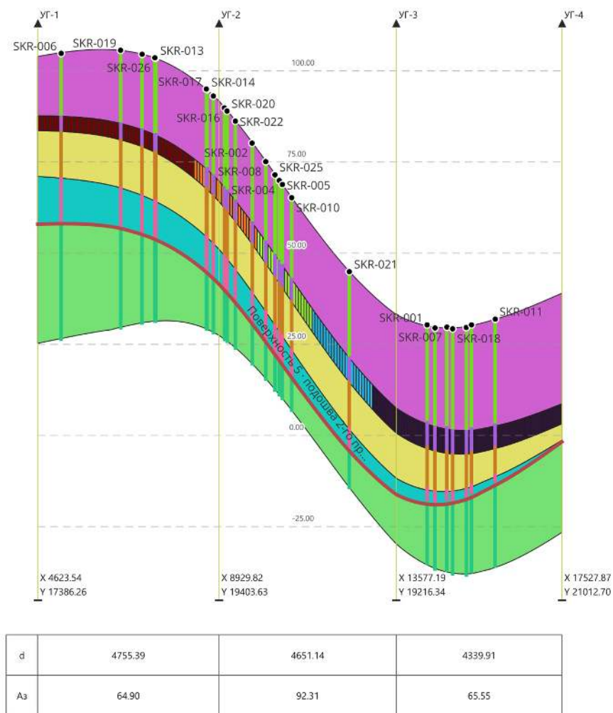
Рис. 39: Оформление разреза: рамка с угловыми вертикалями и треугольниками, горизонтальные оси с отметками слева и таблица углов под разрезом.
