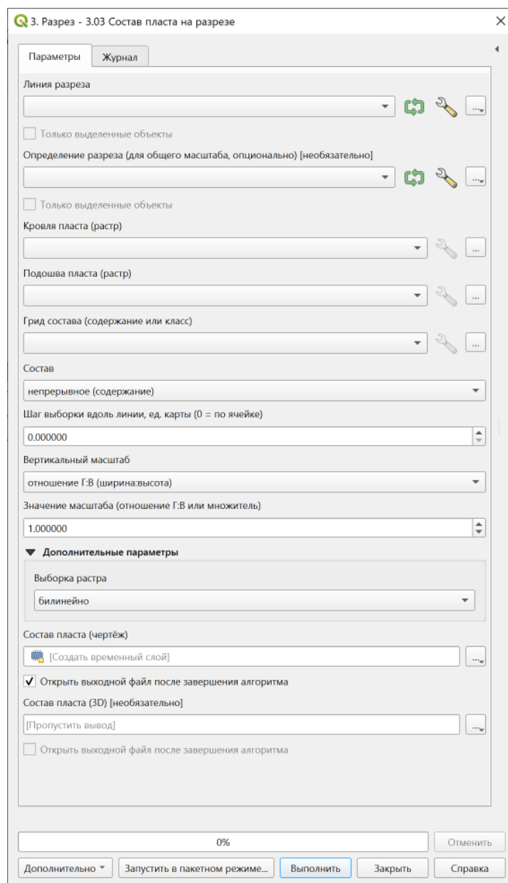
Рис. 38: Окно 3.03: линия, кровля и подошва пласта, грид состава и режим содержание или класс.
