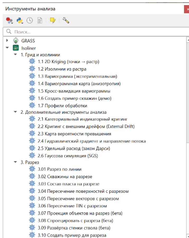
Рис. 1: Инструменты модуля в панели «Обработка»: провайдер Isoliner с тремя группами - «1. Грид и изолинии» (1.1-1.7), «2. Дополнительные инструменты анализа» (2.1-2.6) и «3. Разрез» (3.01-3.10) и «4. Пласт и блочная модель» (4.01-4.04).
