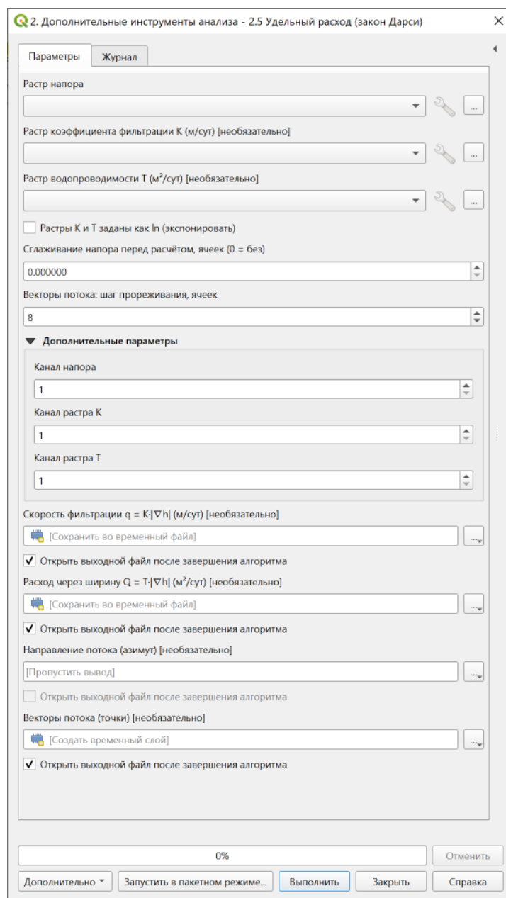
Рис. 33: Окно 2.5: растр напора, растры свойств пласта K/T и выходы скорости, расхода, направления.
