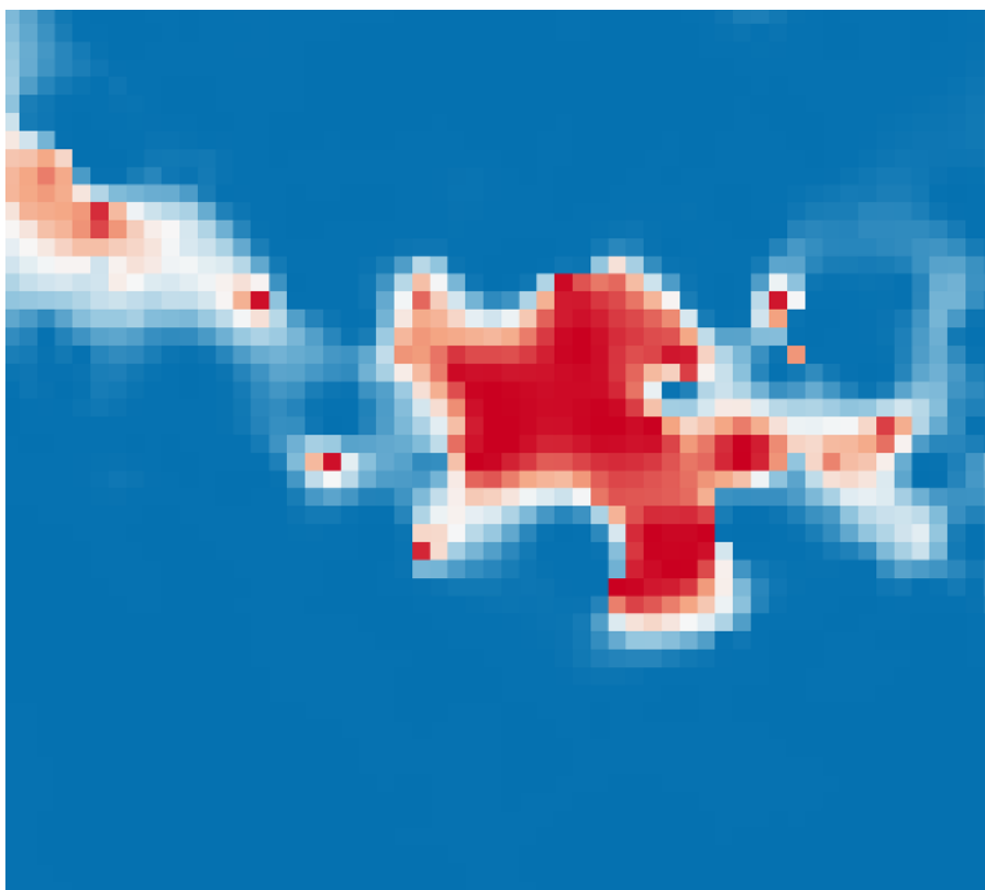
Рис. 31: Карта вероятности превышения с расходящейся шкалой и переломом на 0.5. Красное - значение уверенно выше порога, синее - уверенно ниже, белый поясok по линии P=0.5 - зона неопределённости (спорные значения). Чем дальше от скважин, тем шире поясok.
