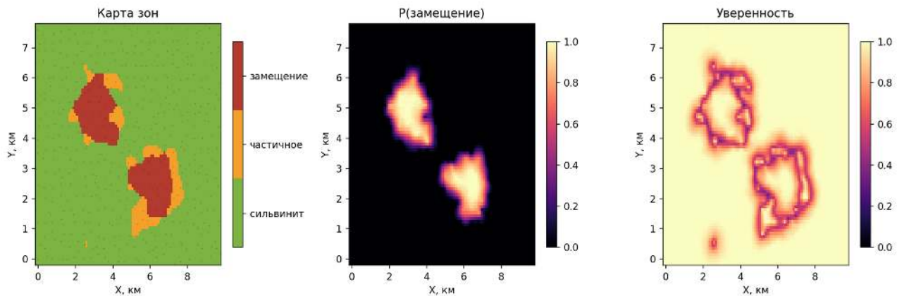
Рис. 26: Категориальный индикаторный кригинг на учебном руднике: карта зон по максимуму вероятности, поверхность вероятности замещения и уверенность. На границах зон уверенность падает.
