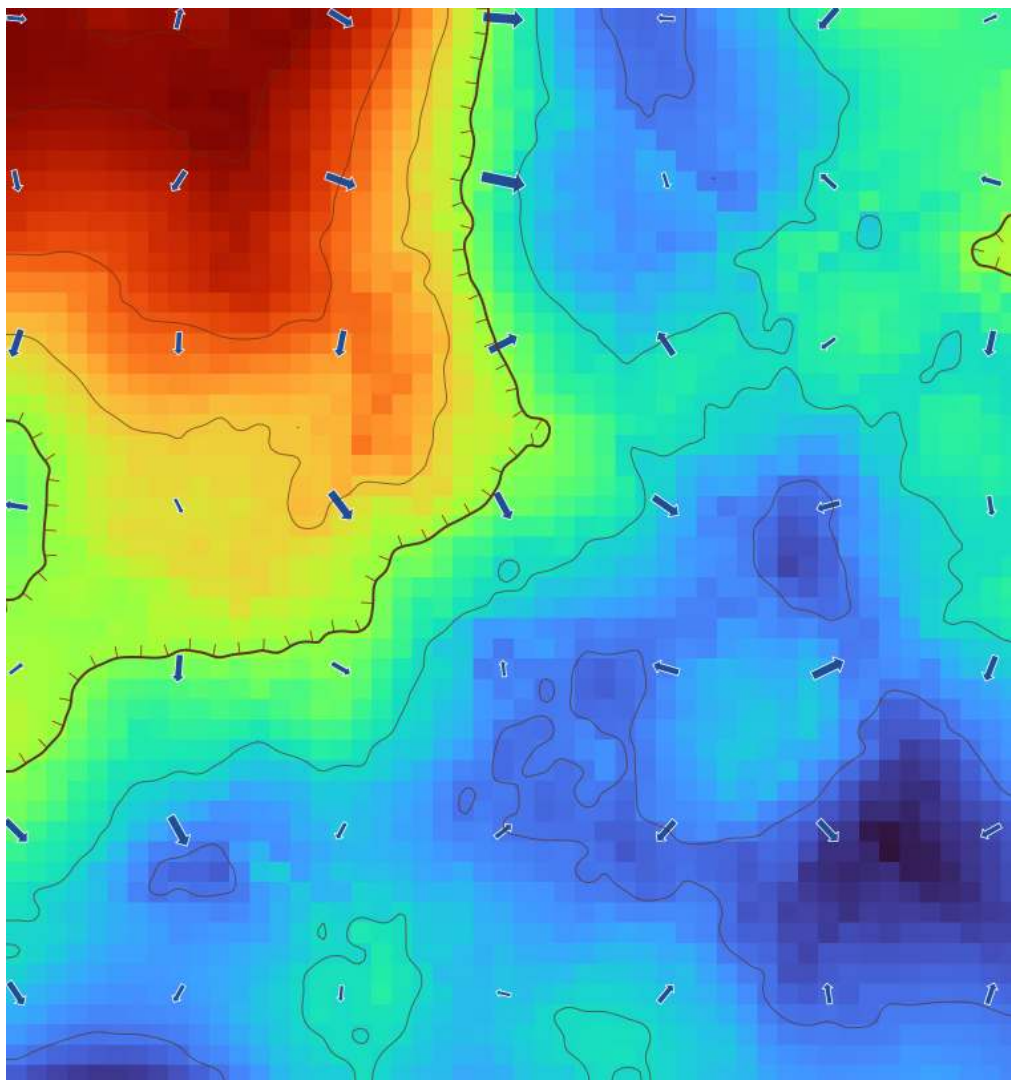
Рис. 30: Векторы потока на поверхности напора: стрелки идут вниз по градиенту, от высокого напора (тёплые тона) к низкому (холодные), поверх изолиний напора. Длина стрелки растёт с крутизной градиента.
