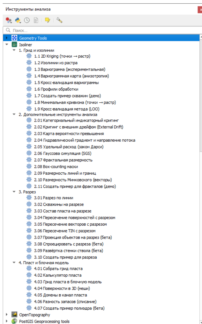
Рис. 1: Провайдер Isoliner в панели «Обработка»: четыре группы, тридцать семь инструментов.
