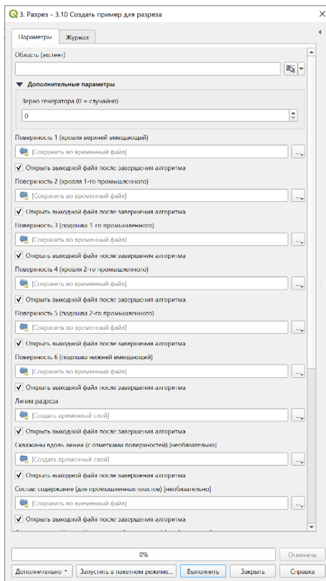
Рис. 49: Окно 3.10: экстенд, шесть поверхностей с подписями кровля/подошва, линия, скважины и гриды состава.
