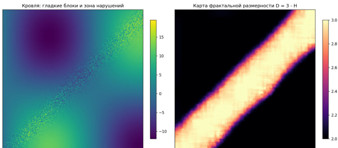
Рис. 38: Синтетическая кровля с диагональной зоной дробления и её карта D: спокойные блоки около 2, зона нарушений проявилась ярким линеamentом.
