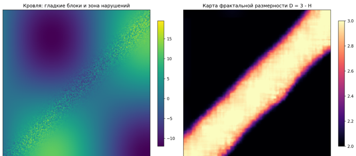
Рис. 31: Синтетическая кровля с диагональной зоной дробления и её карта D: спокойные блоки около 2, зона нарушений проявилась ярким линеamentом.
