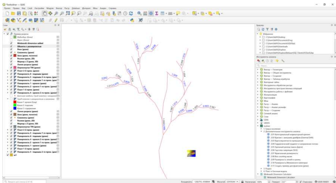
Рис. 33: Демо-реки с подписями D_{\text{mink}} по рукавам: почти гладкие рукава дают значения около единицы, сеть целиком - выше.
