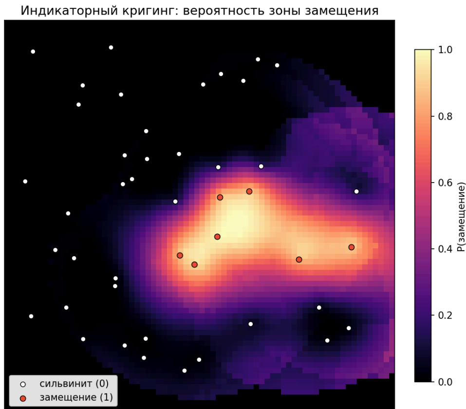
Рис. 22: Индикаторный кригинг на синтетике: скважины с категорией (красные - замещение, белые - сальвинит) превращаются в карту вероятности класса. Порогом 0.5 из неё режется контур домена.
