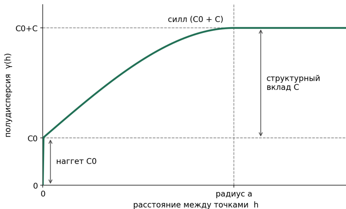
Рис. 5: Схема вариограммы: наггет C_0 , структурный вклад C , sill ( C_0 + C ) и радиус корреляции a .
