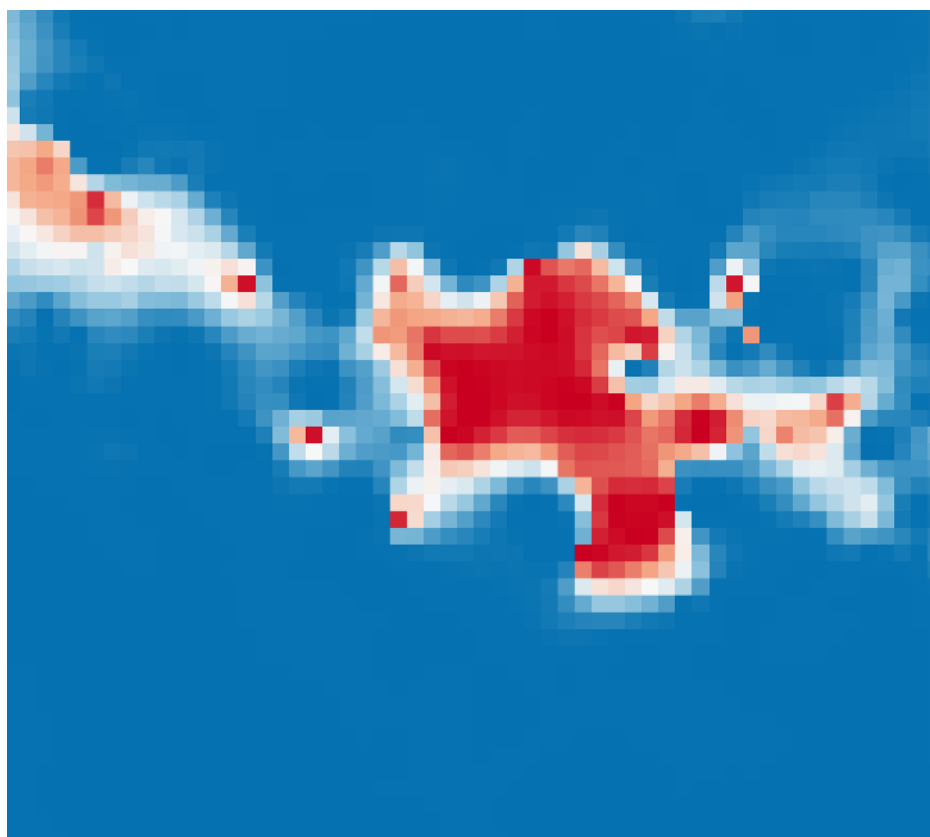
Рис. 26: Карта вероятности превышения с расходящейся шкалой и переломом на 0.5. Красное - значение уверенно выше порога, синее - уверенно ниже, белый поясик по линии P=0.5 - зона неопределённости (спорные значения). Чем дальше от скважин, тем шире поясик.
