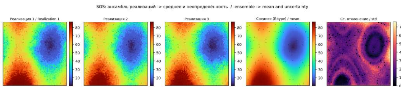
Рис. 40: Ансамбль реализаций SGS и производные от него среднее и неопределённость.
