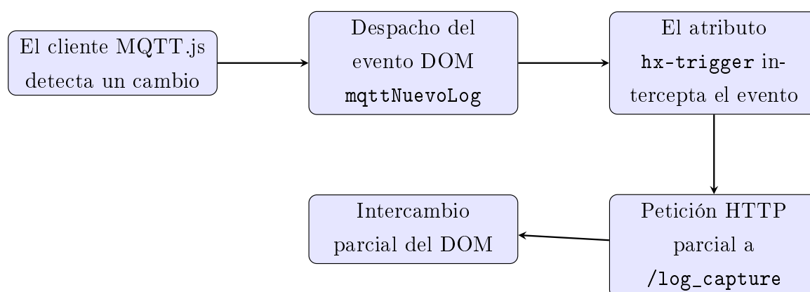
Figura 2.17. Flujo de actualización reactiva del DOM mediante eventos MQTT y atributos HTMX.
