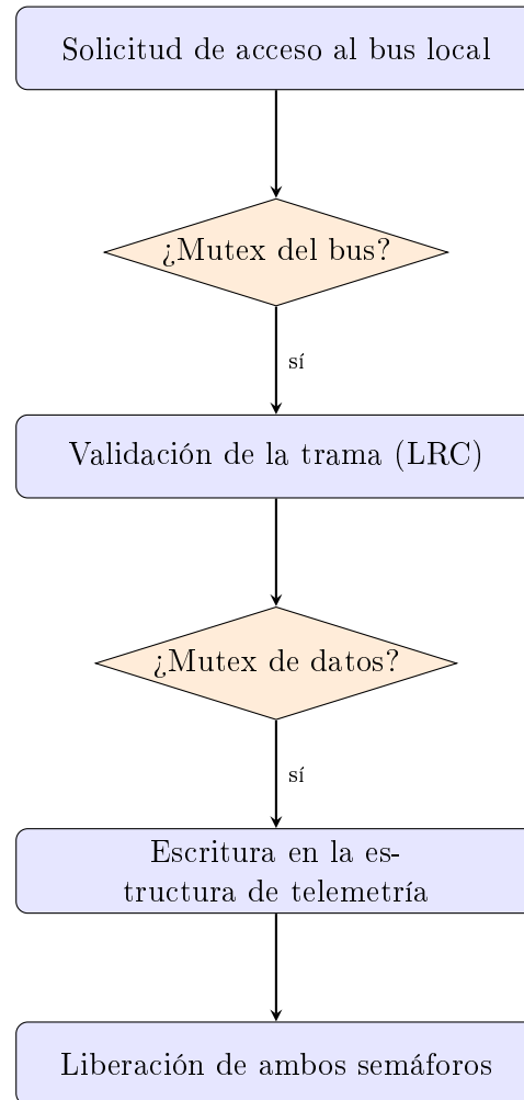
Figura 2.14. Exclusión mutua en dos niveles para la protección de la memoria RAM y del bus físico.
