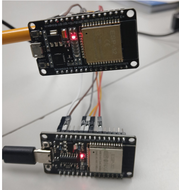
Figura 3.3. Montaje del banco de pruebas Hardware-in-the-Loop: el ESP32 maestro (MT-IoT) y el ESP32 esclavo que emula al periférico fiscal, interconectados sobre el bus síncrono local.
