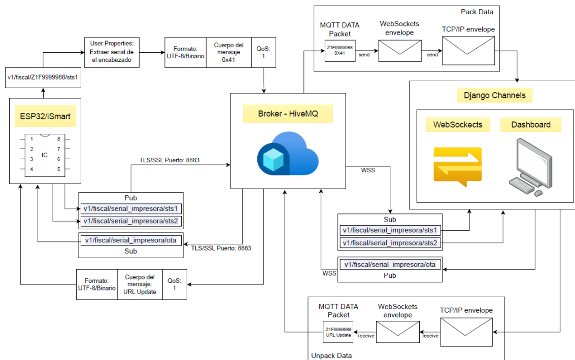
Figura 2.3. Diagrama propuesto para la arquitectura de comunicaciones MQTT.
