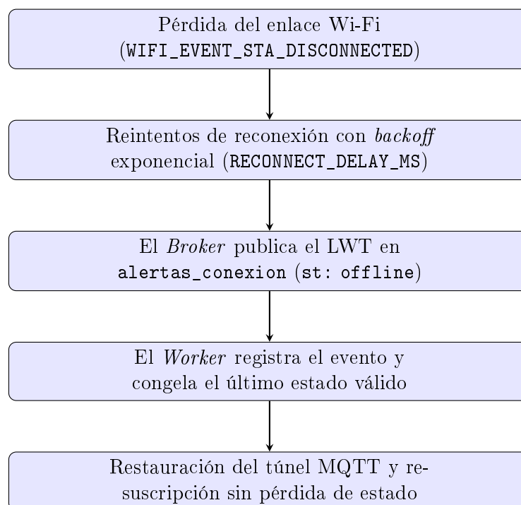
Figura 3.7. Diagrama de flujo de la resiliencia de red y del ciclo de detección, reconexión y restauración del túnel MQTT.
