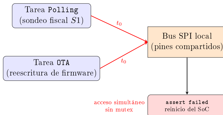
Figura 2.12. Trazo de depuración y registro de evento ante colisión por acceso concurrente al bus local (Choque de Trenes).
