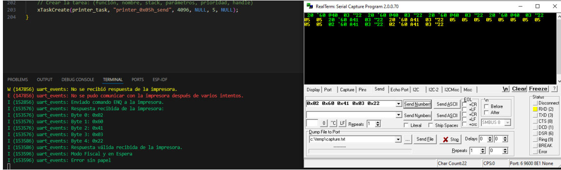
Figura 2.9. Captura de inyección manual de tramas y comando ENQ mediante la terminal de datos RealTerm.
