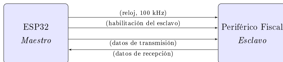
Figura 2.13. Interacción maestro-esclavo sobre el bus síncrono local, con señal de reloj dedicada a 100 kHz y vías independientes de transmisión y recepción.
