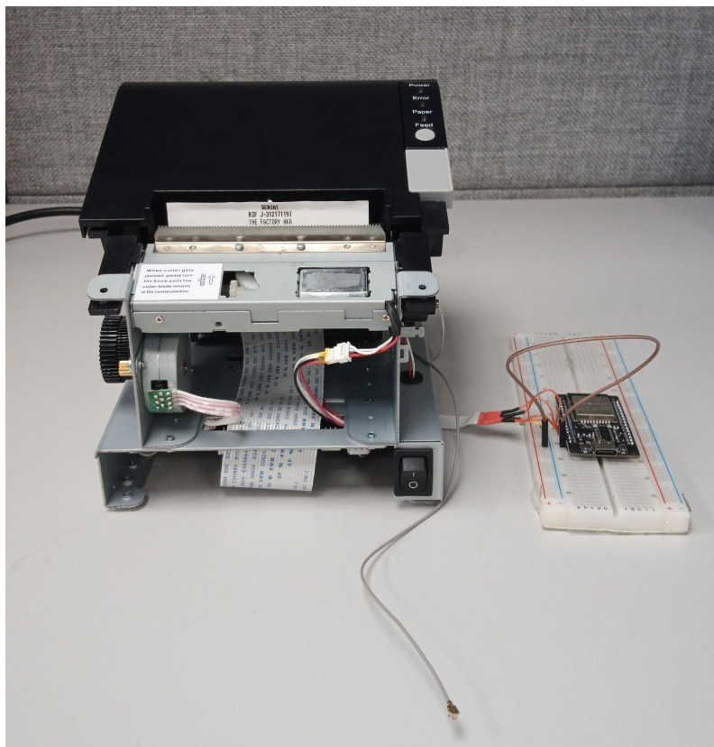
Figura 3.1. Prototipo funcional del MT-IoT integrado a la impresora fiscal en entorno de pruebas.
