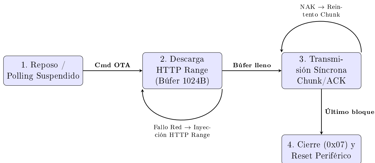
Figura 2.16. Máquina de estados del bridge síncrono para reprogramación de periféricos locales.
