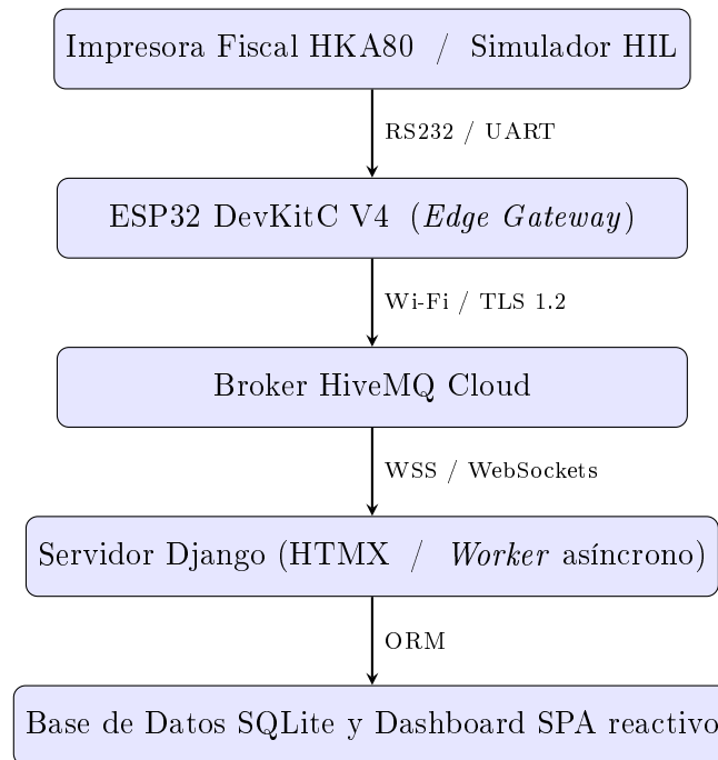
Figura 3.2. Arquitectura IloT definitiva del sistema, desplegada en borde y nube.
