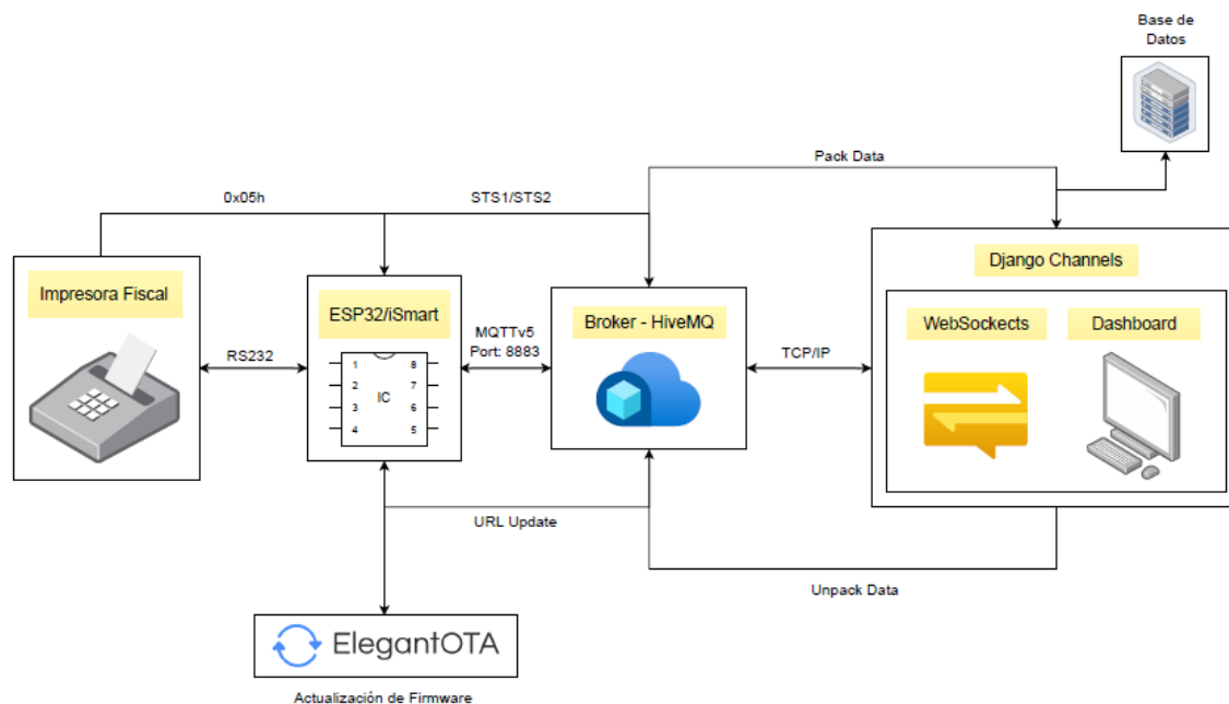
Figura 2.2. Diagrama de la Arquitectura IIoT distribuida en tres niveles (Edge, Gateway y Cloud).
