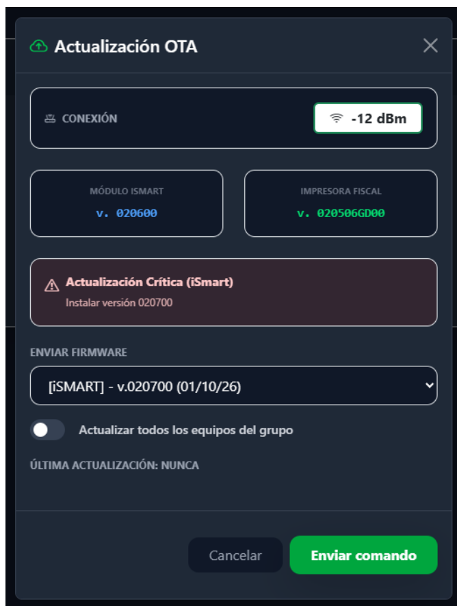
Figura 3.10. Intermediación web desplegando una actualización de firmware crítica hacia el MT-IoT.
