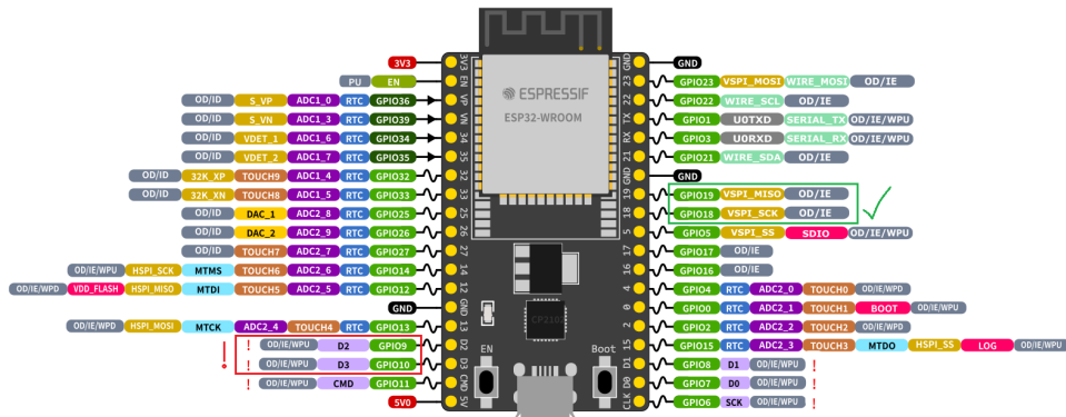
Figura 2.4. Pinlayout de la tarjeta ESP32 DevKitC V4 y reasignación de pines seriales.
