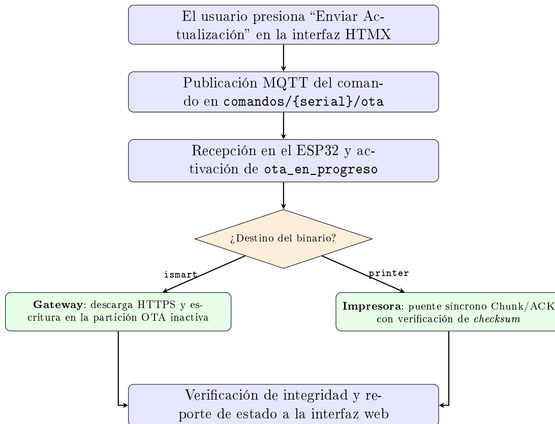
Figura 3.9. Diagrama de flujo de la orquestación de la actualización remota (OTA) de doble objetivo.
