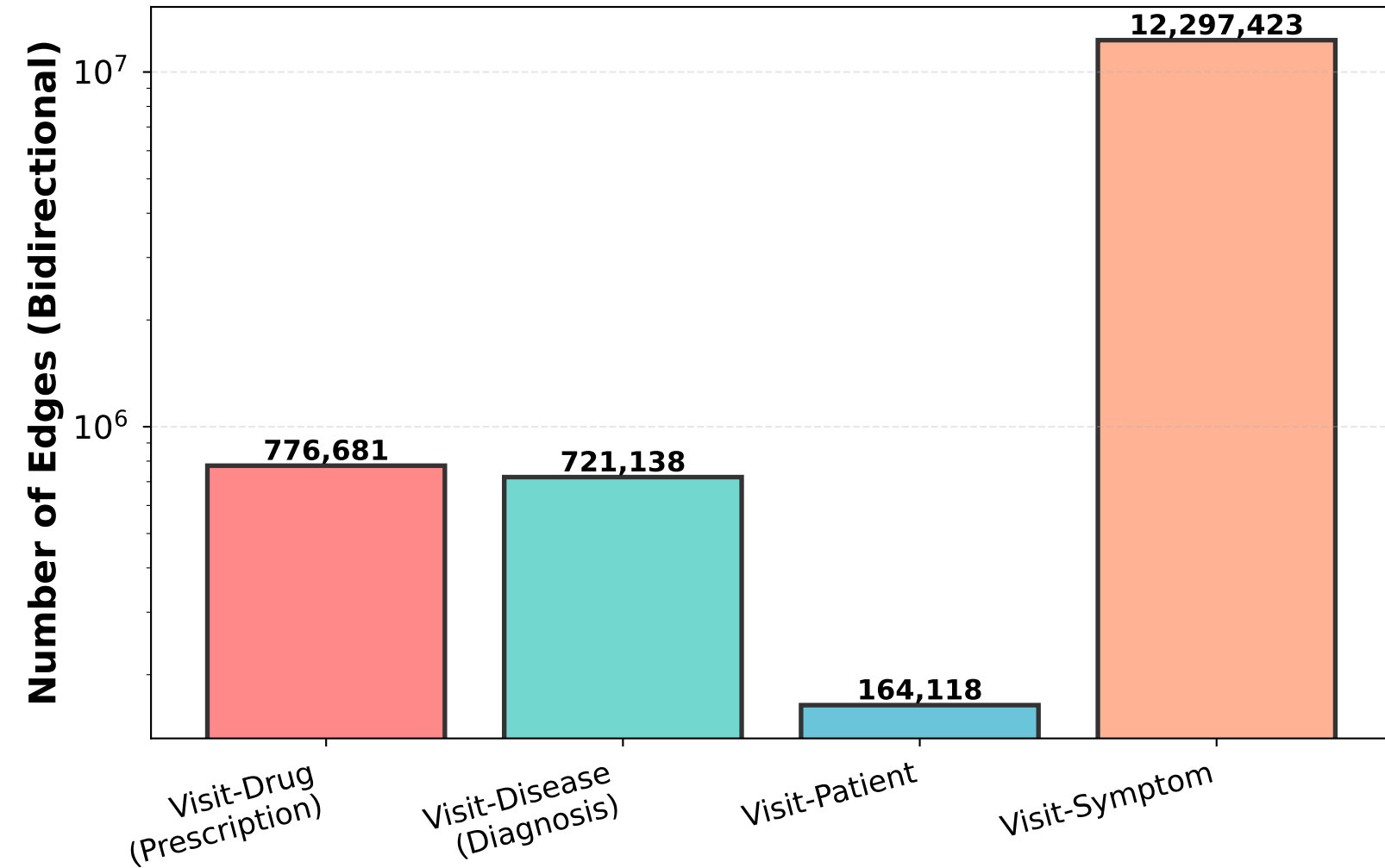
Edge Type Distribution
