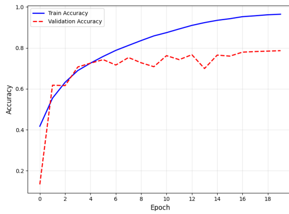
ĐỘ CHÍNH XÁC QUA CÁC EPOCHS
