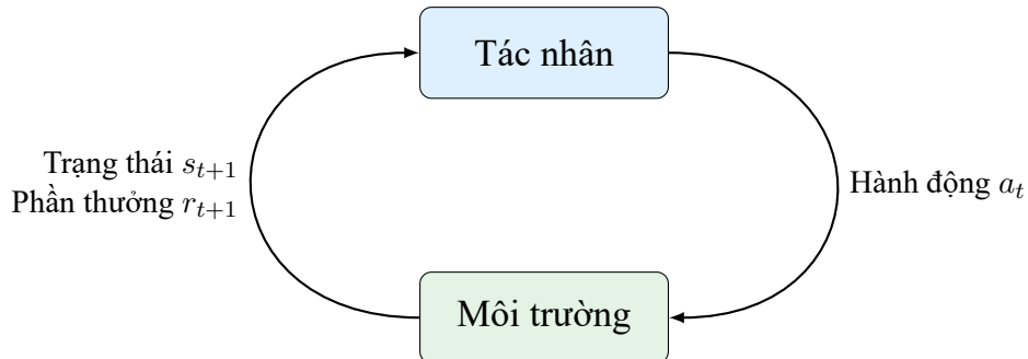
Hình 1.1: Vòng lặp tương tác giữa agent và môi trường trong học tăng cường
