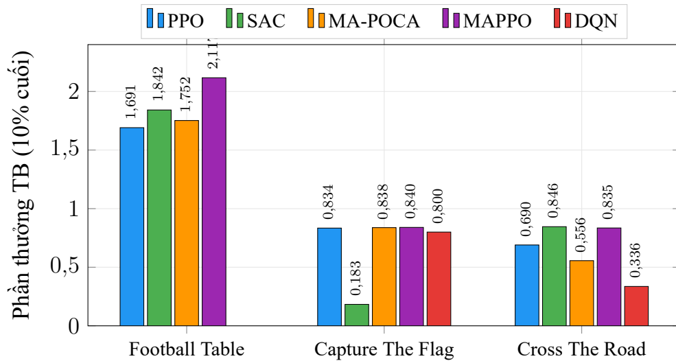
Hình 3.11: Phần thưởng trung bình mười phần trăm cuối của các lần chạy; DQN trên Football Table được loại khỏi biểu đồ vì không dùng self-play
