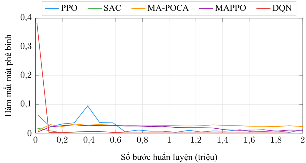
Hình 3.6: Hàm mất mát của mạng phê bình trên môi trường Cross The Road
