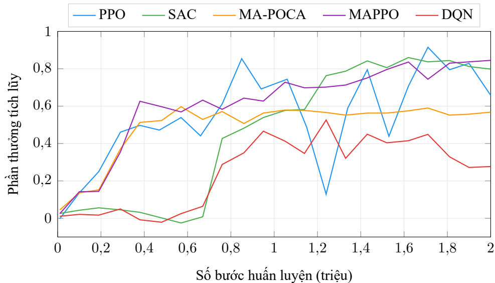
Hình 3.3: Đường cong phần thưởng trên môi trường Cross The Road
