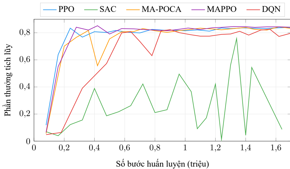
Hình 3.7: Đường cong phần thưởng trên môi trường Capture The Flag
