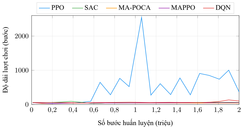
Hình 3.4: Độ dài lượt chơi trên môi trường Cross The Road
