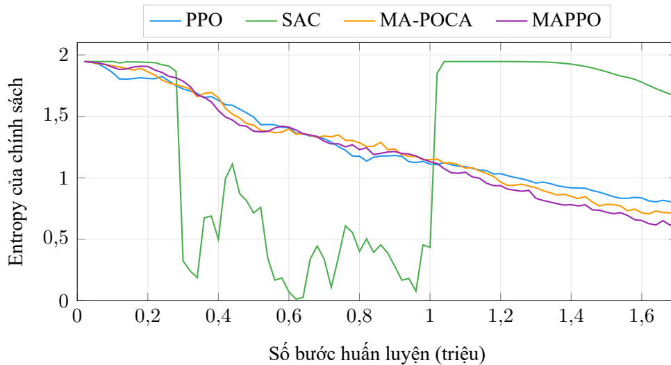
Hình 3.9: Diễn biến entropy của chính sách trên môi trường Capture The Flag: ba thuật toán họ PPO giảm đều, riêng SAC sụp xuống rồi bật ngược về mức cực đại
