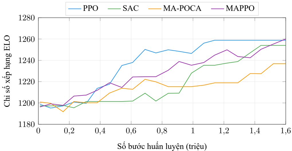
Hình 3.1: Tiến trình chỉ số xếp hạng ELO trong cơ chế tự chơi trên Football Table
