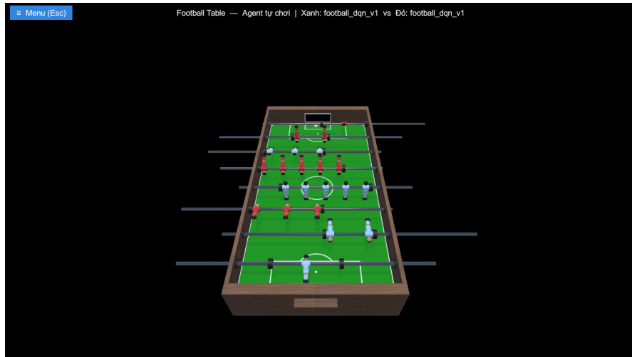
Hình 4.9: Chế độ Agent tự chơi trong Football Table với mô hình football_dqn_v1 : ứng dụng nạp bản scene rời rạc và chỉ giữ lại một bàn trong số tám bàn của cấu hình huấn luyện
