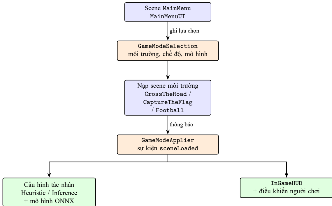
Hình 4.1: Luồng hoạt động của ứng dụng trình diễn
