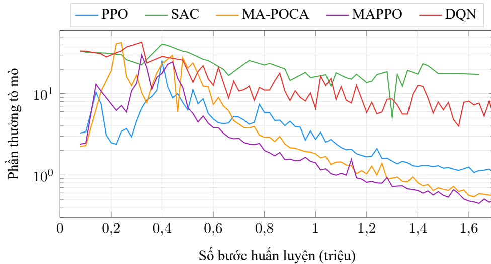
Hình 3.10: Phần thưởng tò mò trên môi trường Capture The Flag (trục tung thang lô-ga-rit)
