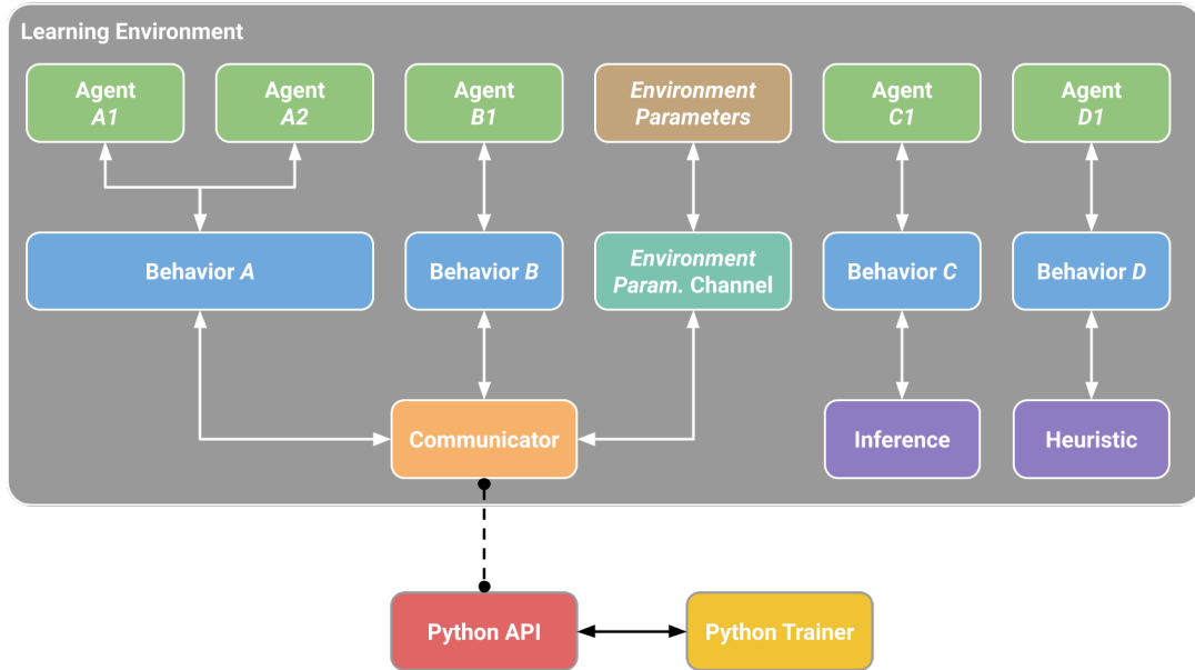
Hình 1.4: Kiến trúc tổng thể của Unity ML-Agents Toolkit
