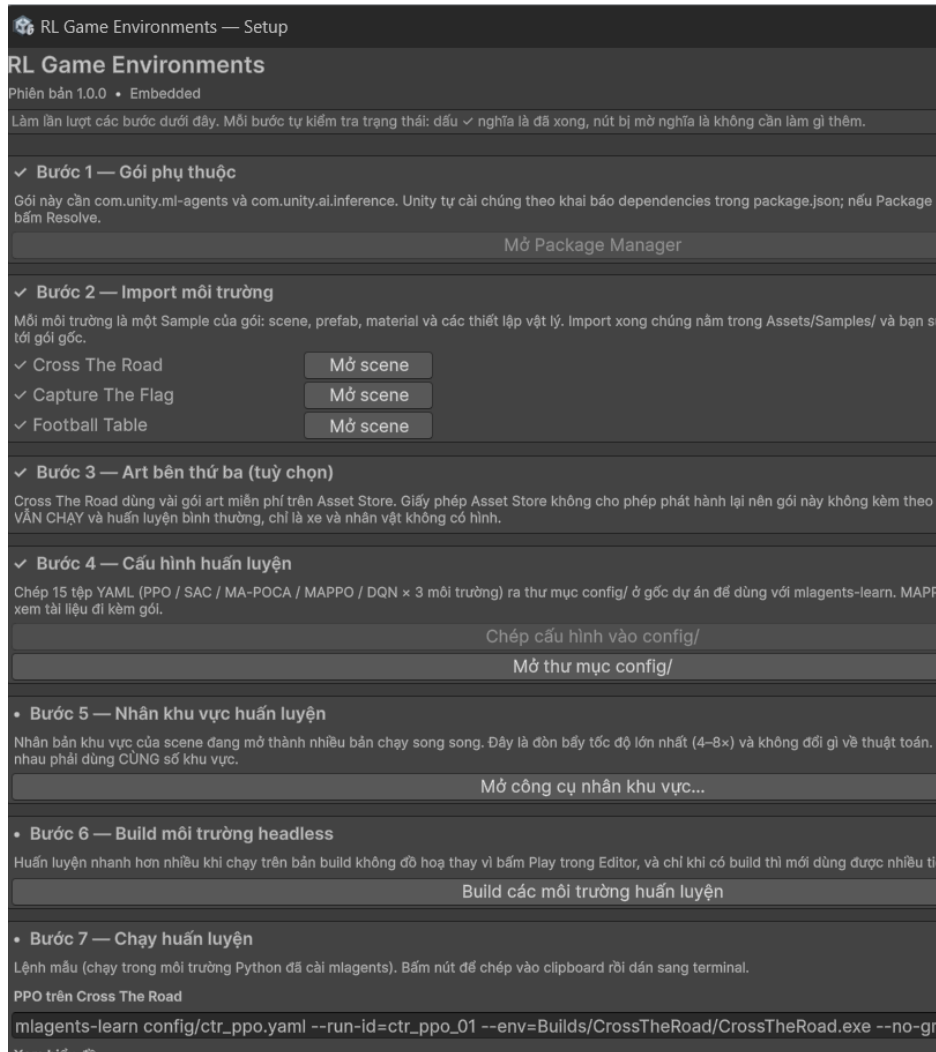
Hình 4.10: Trình hướng dẫn cài đặt của gói: bảy bước, mỗi bước tự kiểm tra trạng thái và chỉ bật nút khi thực sự còn thiếu
