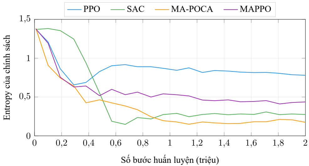
Hình 3.5: Diễn biến entropy của chính sách trên môi trường Cross The Road
