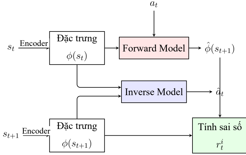
Hình 1.2: Sơ đồ kiến trúc Intrinsic Curiosity Module (ICM)
