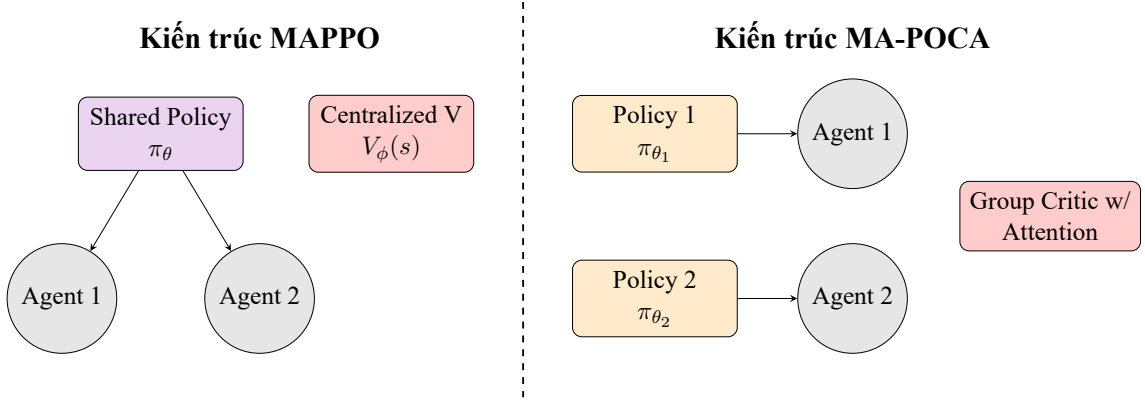
Hình 1.3: So sánh cấu trúc giữa MAPPO và MA-POCA
