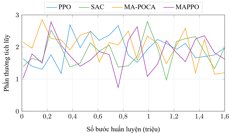
Hình 3.2: Đường cong phần thưởng tích lũy của bốn thuật toán dùng self-play trên môi trường Football Table
