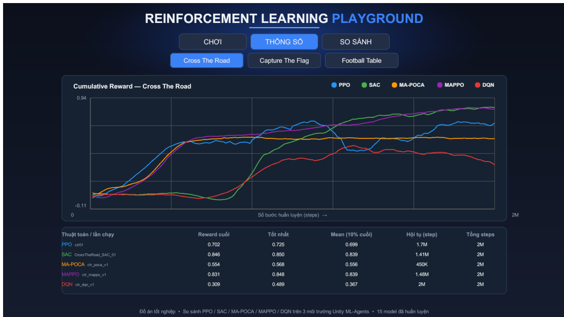
Hình 4.4: Tab THÔNG SỐ: đường cong phần thưởng tích lũy và bảng thống kê của năm thuật toán trên môi trường Cross The Road
