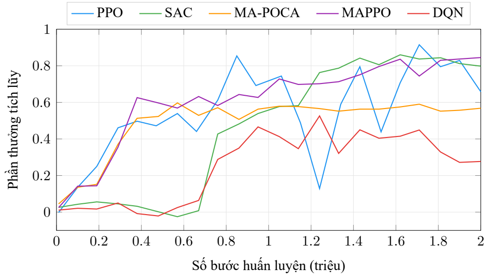
Hình 4.3: Đường cong phần thưởng trên môi trường Cross The Road
