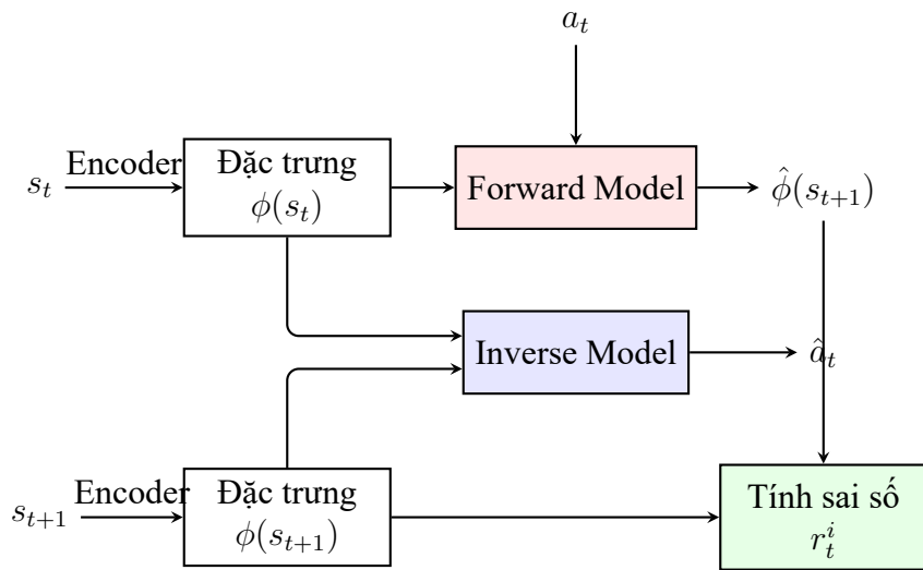
Hình 2.2: Sơ đồ kiến trúc Intrinsic Curiosity Module (ICM)
