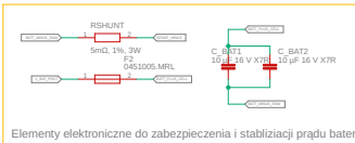
Elementy elektroniczne do zabezpieczenia i stabilizacji prądu baterii
