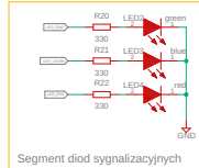
Segment diod sygnalizacyjnych
