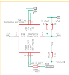
Układ wymuszający prąd 3A USB-C negocjacji
