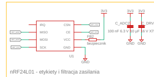
nRF24L01 - etykiety i filtracja zasilania
