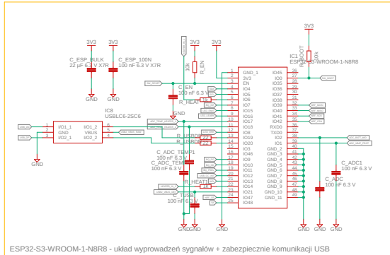
ESP32-S3-WROOM-1-N8R8 - układ wyprowadzeń sygnałów + zabezpieczenie komunikacji USB
