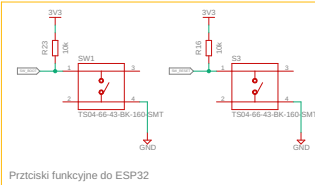
Prztciski funkcyjne do ESP32
