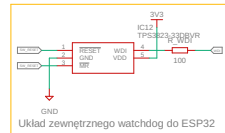
Układ zewnętrznego watchdog do ESP32
