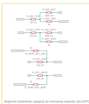
Segment dzielników napięcia do mierzenia wartości dla ESP32
