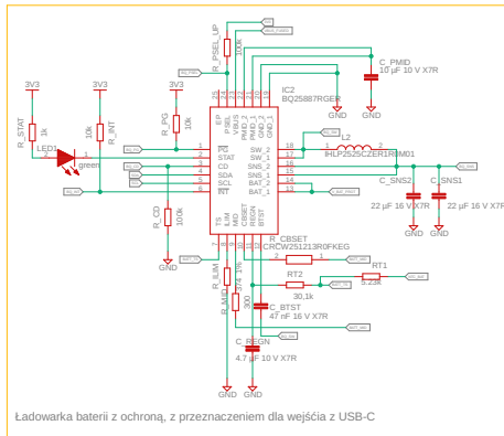
Ładowarka baterii z ochroną, z przeznaczeniem dla wejścia z USB-C
