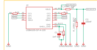
Gniazdo USB-C do komunikacji z ESP32
