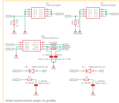
Układysterowania prądu na grzałkę
