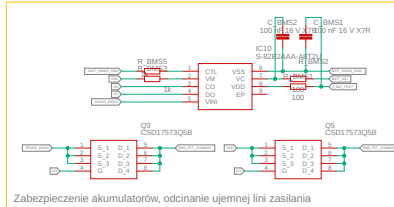
Zabezpieczenie akumulatorów, odcinanie ujemnej linii zasilania
