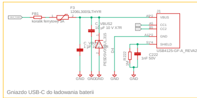
Gniazdo USB-C do ładowania baterii
