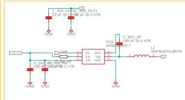
Przetwornica zasilania z Uwyj: 3.3V
