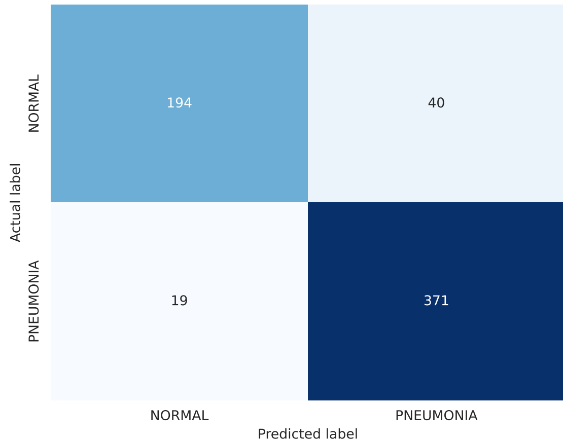
MobileNetV2 -- Confusion Matrix
