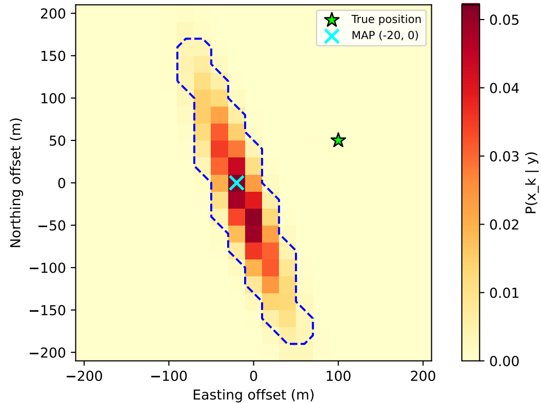
Posterior probability mass over grid
