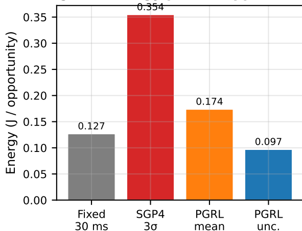
Fig. 3b. Energy per TX Opportunity
