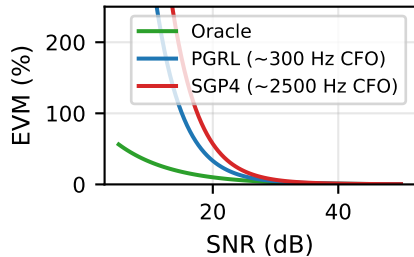
Fig. 5a. EVM vs SNR
