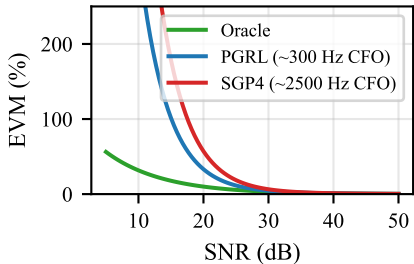
Fig. 5a. EVM vs SNR
