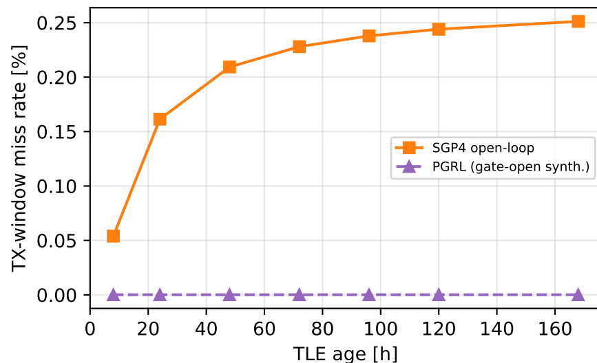
(d) Miss rate vs TLE staleness
