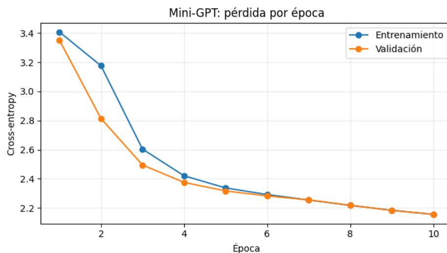
Figura 1. Pérdida de entrenamiento y validación del Mini-GPT por época.
